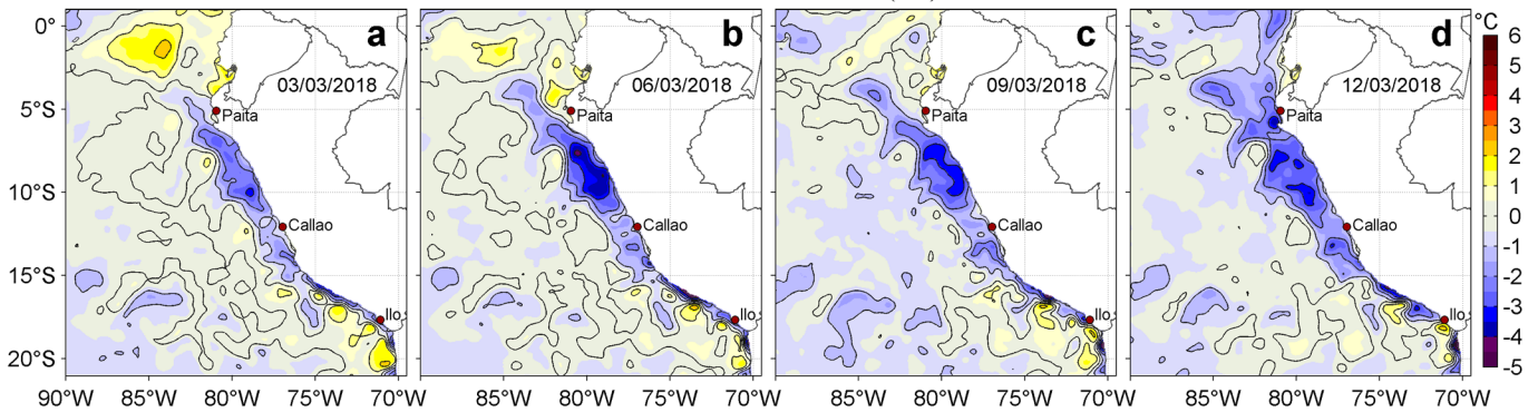
Figura 3. Anomalías de la Temperatura Superficial del Mar ( ^{\circ}\text{C} ) para los días: a) 03, b) 06, c) 09 y d) 12 de marzo de 2018. Las anomalías se calcularon respecto de la climatología para el periodo 2007-2016. Datos: OSTIA-UKMO-L4-GLOB-v2.0 (UK Met Office, 2012; Donlon et al, 2012). Procesamiento: LHF/AFIOF/DGIOCC/IMARPE.
