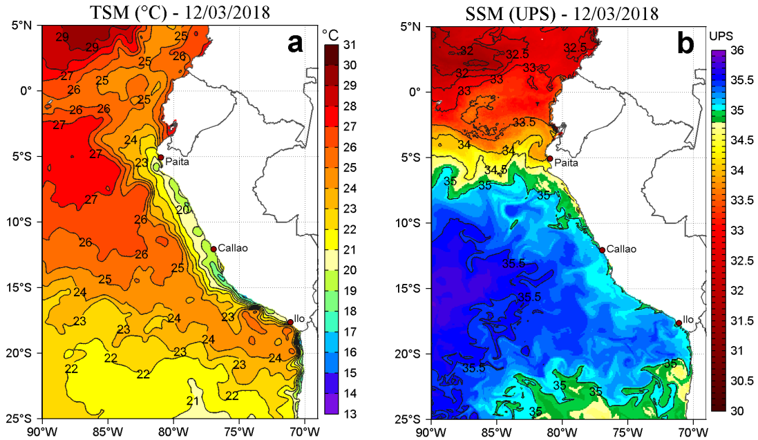
Figura 2. a) Temperatura Superficial del Mar ( ^{\circ}\text{C} ) y b) Salinidad Superficial del Mar (UPS) para el 12 de marzo de 2018. Datos: OSTIA-UKMO-L4-GLOB-v2.0 (UK Met Office, 2012; Donlon et al, 2012) disponible en https://podaac.jpl.nasa.gov/dataset/OSTIA-UKMO-L4-GLOB-v2.0 ) para (a) y Hybrid Coordinate Ocean Model (HYCOM; Halliwell et al., 1998; 2000; Bleck, 2001) para (b). Procesamiento: LHF/AFIOF/DGIOCC/IMARPE.
