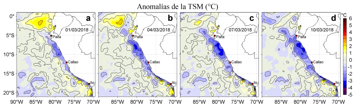
Figura 3. Anomalías de la Temperatura Superficial del Mar ( ^{\circ}\text{C} ) para los días: a) 01, b) 04, c) 07 y d) 10 de marzo de 2018. Las anomalías se calcularon respecto de la climatología para el periodo 2007-2016. Datos: OSTIA-UKMO-L4-GLOB-v2.0 (UK Met Office, 2012; Donlon et al, 2012). Procesamiento: LHF/AFIOF/DGIOCC/IMARPE.
