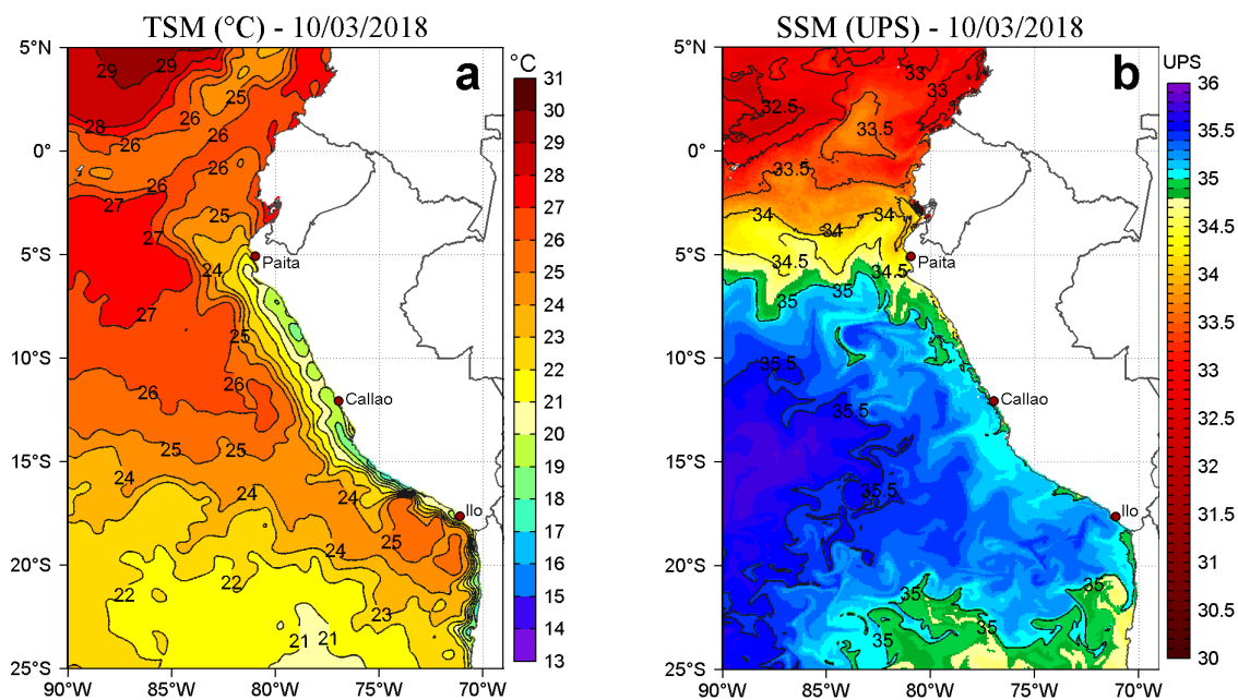
Figura 2. a) Temperatura Superficial del Mar ( ^{\circ}\text{C} ) y b) Salinidad Superficial del Mar (UPS) para el 10 de marzo de 2018. Datos: OSTIA-UKMO-L4-GLOB-v2.0 (UK Met Office, 2012; Donlon et al, 2012) disponible en https://podaac.jpl.nasa.gov/dataset/OSTIA-UKMO-L4-GLOB-v2.0 para (a) y Hybrid Coordinate Ocean Model (HYCOM; Halliwell et al., 1998; 2000; Bleck, 2001) para (b). Procesamiento: LHF/AFIOF/DGIOCC/IMARPE.
