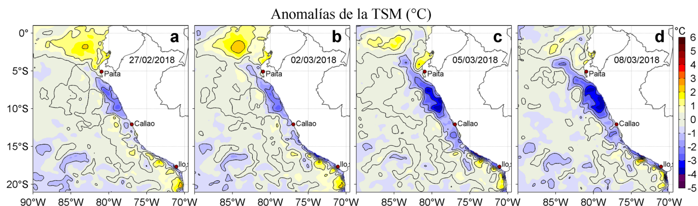
Figura 3. Anomalías de la Temperatura Superficial del Mar ( ^{\circ}\text{C} ) para los días: a) 27 de febrero, b) 02, c) 05 y d) 08 de marzo de 2018. Las anomalías se calcularon respecto de la climatología para el periodo 2007-2016. Datos: OSTIA-UKMO-L4-GLOB-v2.0 (UK Met Office, 2012; Donlon et al, 2012). Procesamiento: LHFM/AFIOF/DGIOCC/IMARPE.
