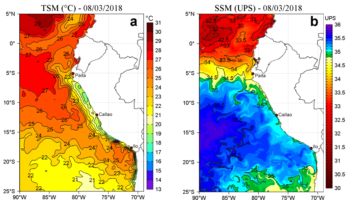
Figura 2. a) Temperatura Superficial del Mar ( ^{\circ}\text{C} ) y b) Salinidad Superficial del Mar (UPS) para el 08 de marzo de 2018. Datos: OSTIA-UKMO-L4-GLOB-v2.0 (UK Met Office, 2012; Donlon et al, 2012) disponible en https://podaac.jpl.nasa.gov/dataset/OSTIA-UKMO-L4-GLOB-v2.0 para (a) y Hybrid Coordinate Ocean Model (HYCOM; Halliwell et al., 1998; 2000; Bleck, 2001) para (b). Procesamiento: LHFM/AFIOF/DGIOCC/IMARPE.
