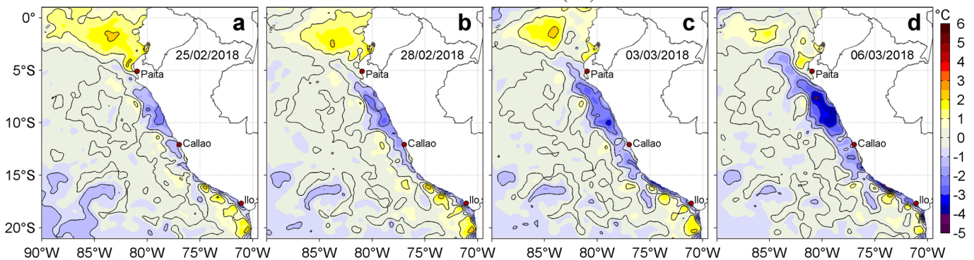
Figura 3. Anomalías de la Temperatura Superficial del Mar (°C) para los días: a) 25, b) 28 de febrero, c) 03 y d) 06 de marzo de 2018. Las anomalías se calcularon respecto de la climatología para el periodo 2007-2016. Datos: OSTIA-UKMO-L4-GLOB-v2.0 (UK Met Office, 2012; Donlon et al, 2012). Procesamiento: LHFM/AFIOF/DGIOCC/IMARPE.
