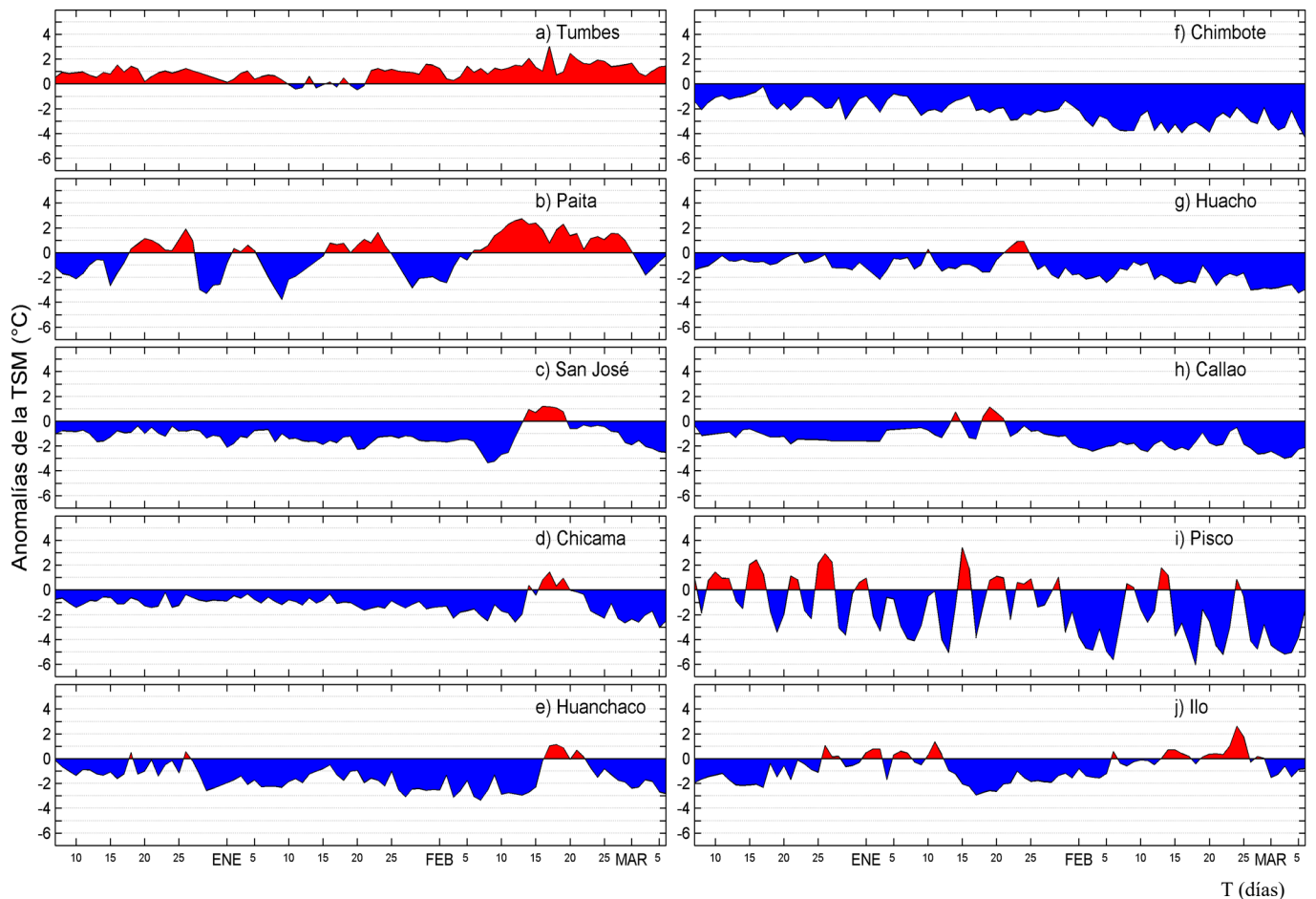
Figura 5. Variación del promedio diario de las anomalías de la Temperatura Superficial del Mar (°C) en la red de estaciones costeras que administra IMARPE en el litoral peruano durante el último trimestre. Las anomalías se calcularon respecto del promedio climatológico pentadal (5 días) para el periodo que se indica en la Tabla 1. Datos y procesamiento: LHF/M/AFIOF/DGIOCC/IMARPE.
