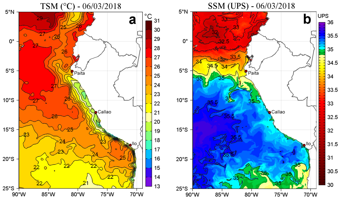
Figura 2. a) Temperatura Superficial del Mar (°C) y b) Salinidad Superficial del Mar (UPS) para el 06 de marzo de 2018. Datos: OSTIA-UKMO-L4-GLOB-v2.0 (UK Met Office, 2012; Donlon et al, 2012) disponible en https://podaac.jpl.nasa.gov/dataset/OSTIA-UKMO-L4-GLOB-v2.0 para (a) y Hybrid Coordinate Ocean Model (HYCOM; Halliwell et al., 1998; 2000; Bleck, 2001) para (b). Procesamiento: LHFM/AFIOF/DGIOCC/IMARPE.
