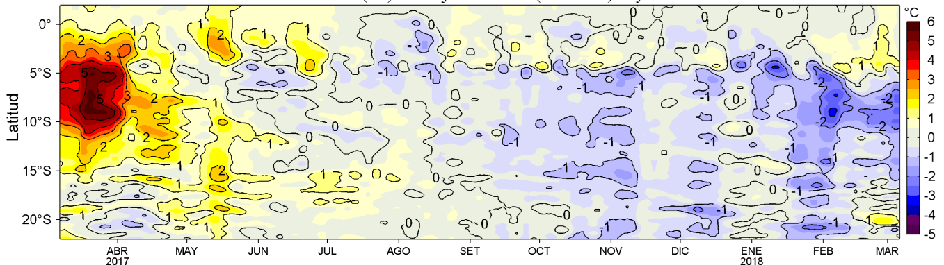
Figura 4. Variación promedio de las anomalías de la Temperatura Superficial del Mar (°C) para una franja de 60 mn (~111 km) adyacente al litoral peruano para los últimos doce meses al 06 de marzo de 2018. Datos: OSTIA-UKMO-L4-GLOB-v2.0 (UK Met. Office, 2012; Donlon et al, 2012) disponible en https://podaac.jpl.nasa.gov/dataset/OSTIA-UKMO-L4-GLOB-v2.0 . Las anomalías se calcularon con respecto al periodo 2007-2016. Procesamiento: LHFM/AFIOF/DGIOCC/IMARPE.
