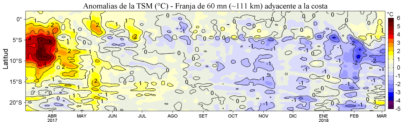
Figura 4. Variación promedio de las anomalías de la Temperatura Superficial del Mar (°C) para una franja de 60 mn (~111 km) adyacente al litoral peruano para los últimos doce meses al 04 de marzo de 2018. Datos: OSTIA-UKMO-L4-GLOB-v2.0 (UK Met. Office, 2012; Donlon et al, 2012) disponible en https://podaac.jpl.nasa.gov/dataset/OSTIA-UKMO-L4-GLOB-v2.0 . Las anomalías se calcularon con respecto al periodo 2007-2016. Procesamiento: LHF/AFIOF/DGIOCC/IMARPE.
