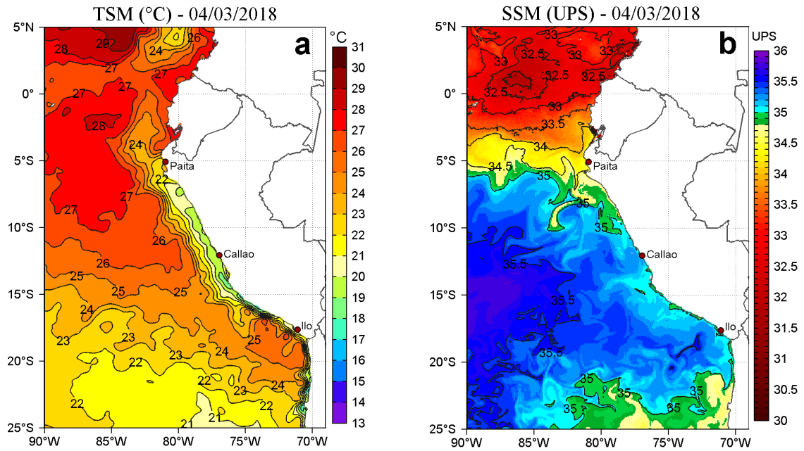
Figura 2. a) Temperatura Superficial del Mar (°C) y b) Salinidad Superficial del Mar (UPS) para el 04 de marzo de 2018. Datos: OSTIA-UKMO-L4-GLOB-v2.0 (UK Met Office, 2012; Donlon et al, 2012) disponible en https://podaac.jpl.nasa.gov/dataset/OSTIA-UKMO-L4-GLOB-v2.0 para (a) y Hybrid Coordinate Ocean Model (HYCOM; Halliwell et al., 1998; 2000; Bleck, 2001) para (b). Procesamiento: LHF/AFIOF/DGIOCC/IMARPE.
