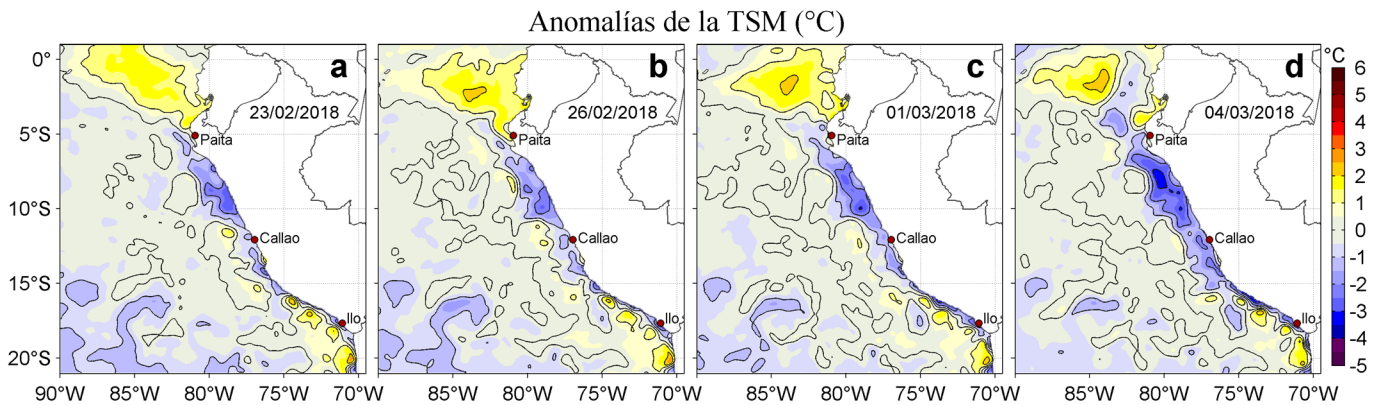
Figura 3. Anomalías de la Temperatura Superficial del Mar (°C) para los días: a) 23, b) 26 de febrero, c) 01 y d) 04 de marzo de 2018. Las anomalías se calcularon respecto de la climatología para el periodo 2007-2016. Datos: OSTIA-UKMO-L4-GLOB-v2.0 (UK Met Office, 2012; Donlon et al, 2012). Procesamiento: LHF/AFIOF/DGIOCC/IMARPE.
