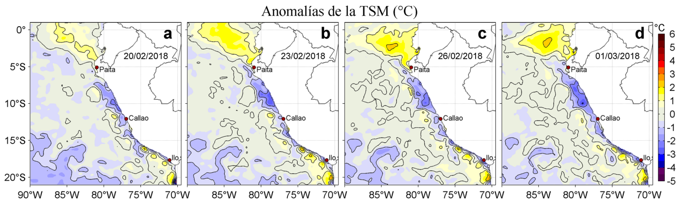
Figura 3. Anomalías de la Temperatura Superficial del Mar ( ^{\circ}\text{C} ) para los días: a) 20, b) 23, c) 26 de febrero y d) 01 de marzo de 2018. Las anomalías se calcularon respecto de la climatología para el periodo 2007-2016. Datos: OSTIA-UKMO-L4-GLOB-v2.0 (UK Met Office, 2012; Donlon et al, 2012). Procesamiento: LHF/AFIOF/DGIOCC/IMARPE.
