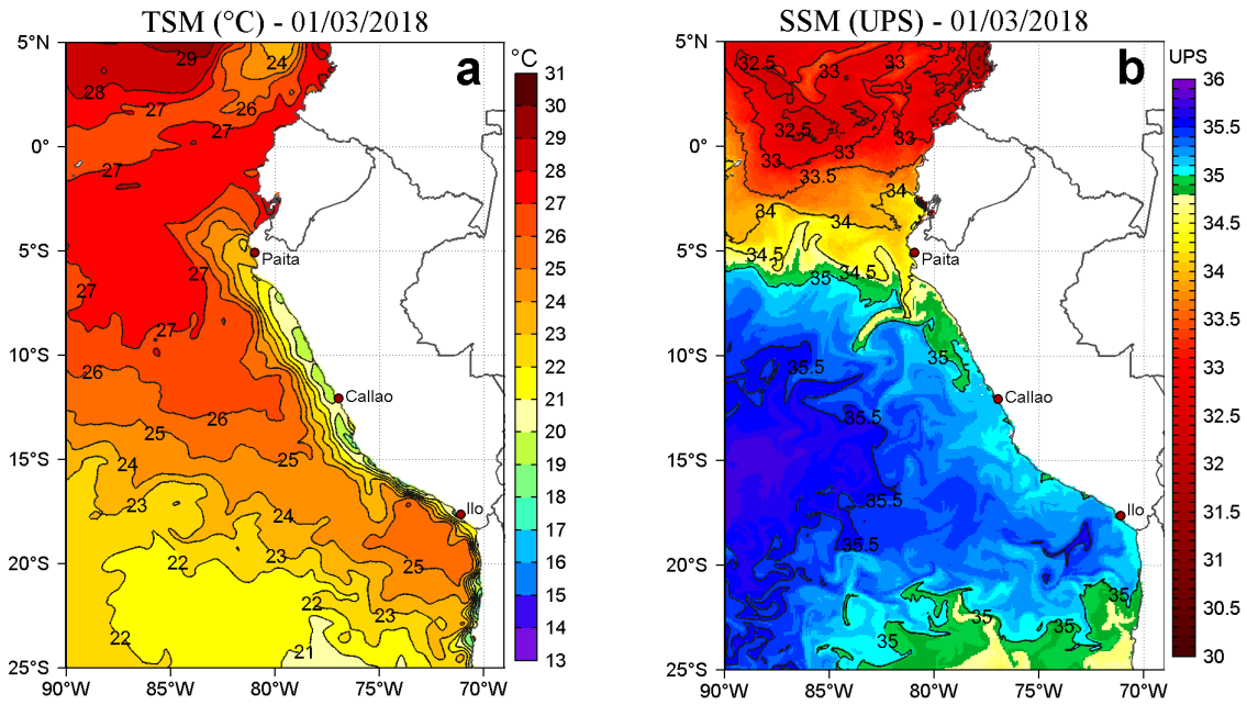
Figura 2. a) Temperatura Superficial del Mar ( ^{\circ}\text{C} ) y b) Salinidad Superficial del Mar (UPS) para el 01 de marzo de 2018. Datos: OSTIA-UKMO-L4-GLOB-v2.0 (UK Met Office, 2012; Donlon et al, 2012) disponible en https://podaac.jpl.nasa.gov/dataset/OSTIA-UKMO-L4-GLOB-v2.0 para (a) y Hybrid Coordinate Ocean Model (HYCOM; Halliwell et al., 1998; 2000; Bleck, 2001) para (b). Procesamiento: LHF/AFIOF/DGIOCC/IMARPE.
