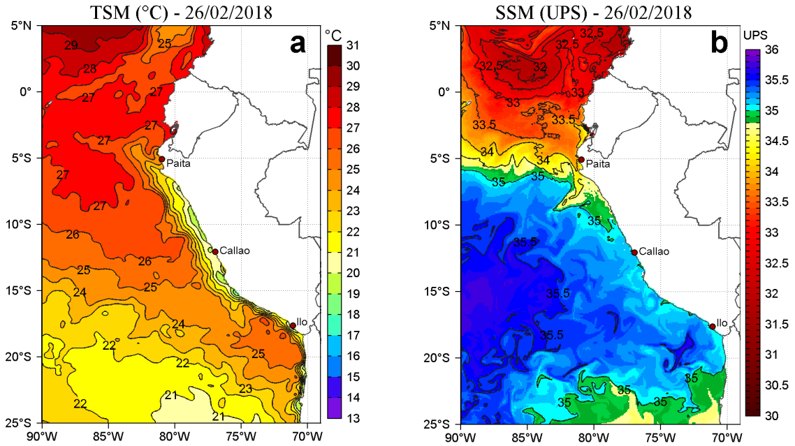
Figura 2. a) Temperatura Superficial del Mar (°C) y b) Salinidad Superficial del Mar (UPS) para el 26 de febrero de 2018. Datos: OSTIA-UKMO-L4-GLOB-v2.0 (UK Met Office, 2012; Donlon et al, 2012) disponible en https://podaac.jpl.nasa.gov/dataset/OSTIA-UKMO-L4-GLOB-v2.0 para (a) y Hybrid Coordinate Ocean Model (HYCOM; Halliwell et al., 1998; 2000; Bleck, 2001) para (b). Procesamiento: LHF/AFIOF/DGIOCC/IMARPE.
