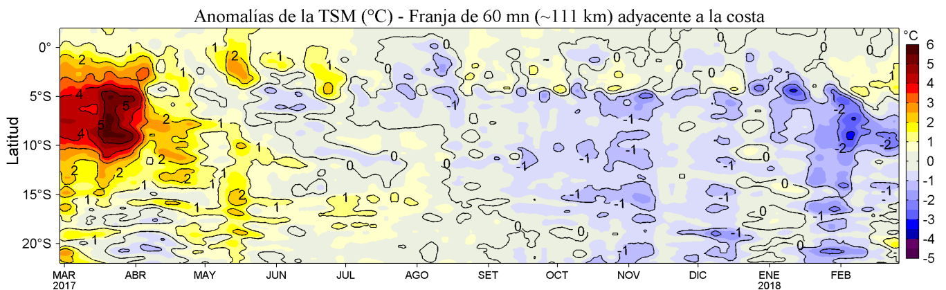
Figura 4. Variación promedio de las anomalías de la Temperatura Superficial del Mar (°C) para una franja de 60 mn (~111 km) adyacente al litoral peruano para los últimos doce meses al 26 de febrero de 2018. Datos: OSTIA-UKMO-L4-GLOB-v2.0 (UK Met. Office, 2012; Donlon et al, 2012) disponible en https://podaac.jpl.nasa.gov/dataset/OSTIA-UKMO-L4-GLOB-v2.0 . Las anomalías se calcularon con respecto al periodo 2007-2016. Procesamiento: LHF/AFIOF/DGIOCC/IMARPE.
