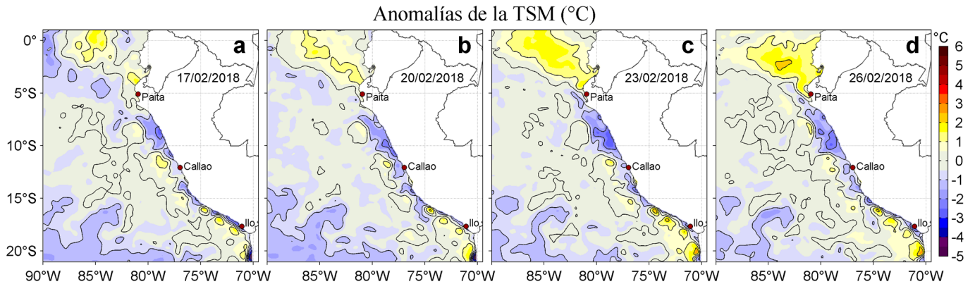
Figura 3. Anomalías de la Temperatura Superficial del Mar (°C) para los días: a) 17, b) 20, c) 23 y d) 26 de febrero de 2018. Las anomalías se calcularon respecto de la climatología para el periodo 2007-2016. Datos: OSTIA-UKMO-L4-GLOB-v2.0 (UK Met Office, 2012; Donlon et al, 2012). Procesamiento: LHF/AFIOF/DGIOCC/IMARPE.
