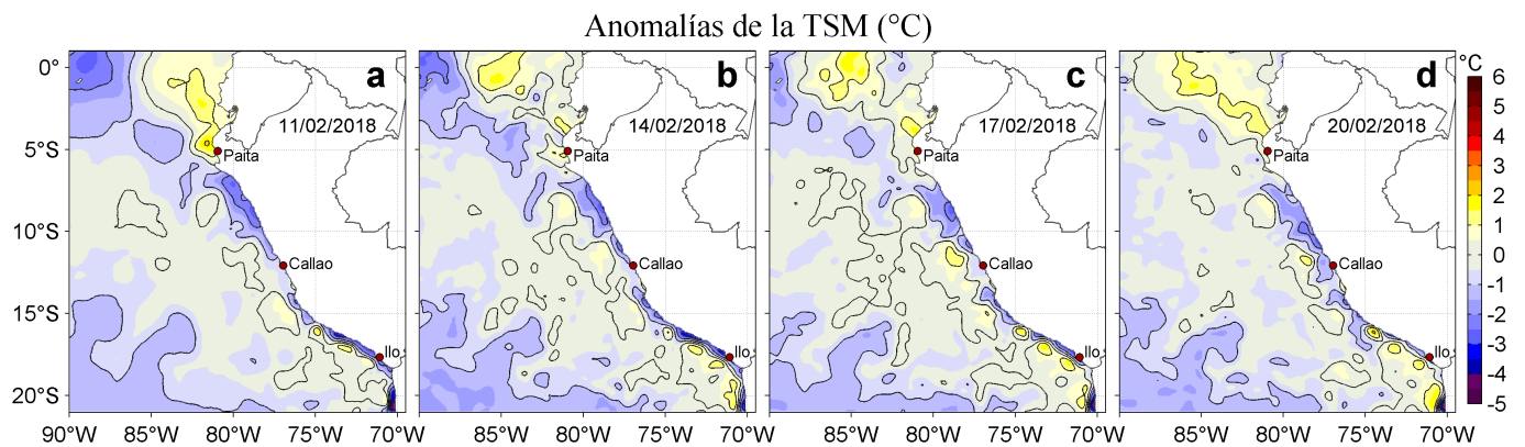
Figura 3. Anomalías de la Temperatura Superficial del Mar ( ^{\circ}\text{C} ) para los días: a) 11, b) 14, c) 17 y d) 20 de febrero de 2018. Las anomalías se calcularon respecto de la climatología para el periodo 2007-2016. Datos: OSTIA-UKMO-L4-GLOB-v2.0 (UK Met Office, 2012; Donlon et al, 2012). Procesamiento: LHF/AFIOF/DGIOCC/IMARPE.
