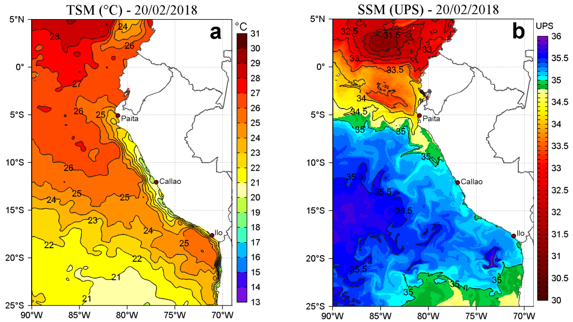
Figura 2. a) Temperatura superficial del mar ( ^{\circ}\text{C} ) y b) Salinidad superficial del mar (UPS) para el 20 de febrero de 2018. Datos: OSTIA-UKMO-L4-GLOB-v2.0 (UK Met Office, 2012; Donlon et al, 2012) disponible en https://podaac.jpl.nasa.gov/dataset/OSTIA-UKMO-L4-GLOB-v2.0 para (a) y Hybrid Coordinate Ocean Model (HYCOM; Halliwell et al., 1998; 2000; Bleck, 2001) para (b). Procesamiento: LHF/AFIOF/DGIOCC/IMARPE.
