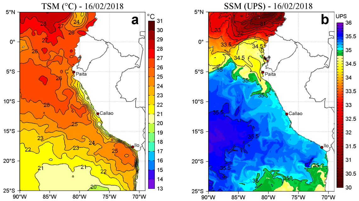
Figura 2. a) Temperatura superficial del mar ( ^{\circ}\text{C} ) y b) Salinidad superficial del mar (UPS) para el 16 de febrero de 2018. Datos: OSTIA-UKMO-L4-GLOB-v2.0 (UK Met Office, 2012; Donlon et al., 2012) disponible en https://podaac.jpl.nasa.gov/dataset/OSTIA-UKMO-L4-GLOB-v2.0 para (a) y Hybrid Coordinate Ocean Model (HYCOM; Halliwell et al., 1998; 2000; Bleck, 2001) para (b). Procesamiento: LHFM/AFIOF/DGIOCC/IMARPE.
