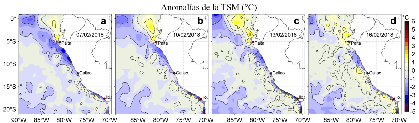
Figura 3. Anomalías de la Temperatura Superficial del Mar ( ^{\circ}\text{C} ) para los días: a) 07, b) 10, c) 13 y d) 16 de febrero de 2018. Las anomalías se calcularon respecto de la climatología para el periodo 2007-2016. Datos: OSTIA-UKMO-L4-GLOB-v2.0 (UK Met Office, 2012; Donlon et al., 2012). Procesamiento: LHFM/AFIOF/DGIOCC/IMARPE.
