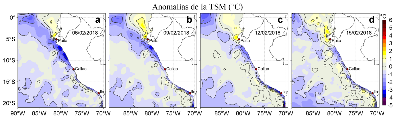
Figura 3. Anomalías de la Temperatura Superficial del Mar ( ^{\circ}\text{C} ) para los días: a) 06, b) 09, c) 12 y d) 15 de febrero de 2018. Las anomalías se calcularon respecto de la climatología para el periodo 2007-2016. Datos: OSTIA-UKMO-L4-GLOB-v2.0 (UK Met Office, 2012; Donlon et al, 2012). Procesamiento: LHF/AFIOF/DGIOCC/IMARPE.
