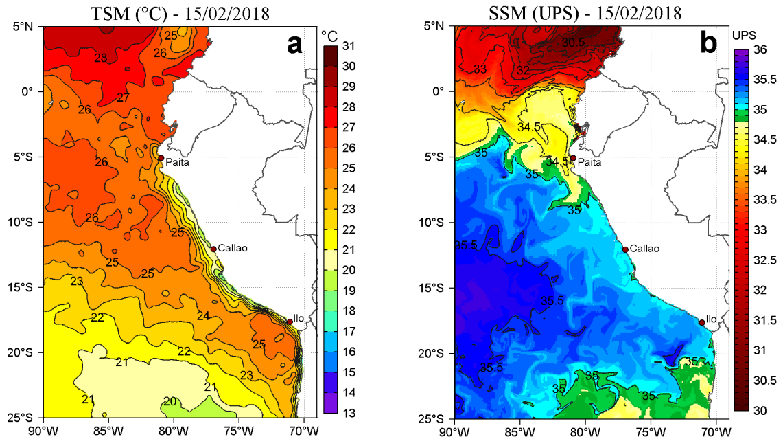
Figura 2. a) Temperatura superficial del mar ( ^{\circ}\text{C} ) y b) Salinidad superficial del mar (UPS) para el 15 de febrero de 2018. Datos: OSTIA-UKMO-L4-GLOB-v2.0 (UK Met Office, 2012; Donlon et al, 2012) disponible en https://podaac.jpl.nasa.gov/dataset/OSTIA-UKMO-L4-GLOB-v2.0 para (a) y Hybrid Coordinate Ocean Model (HYCOM; Halliwell et al., 1998; 2000; Bleck, 2001) para (b). Procesamiento: LHF/AFIOF/DGIOCC/IMARPE.
