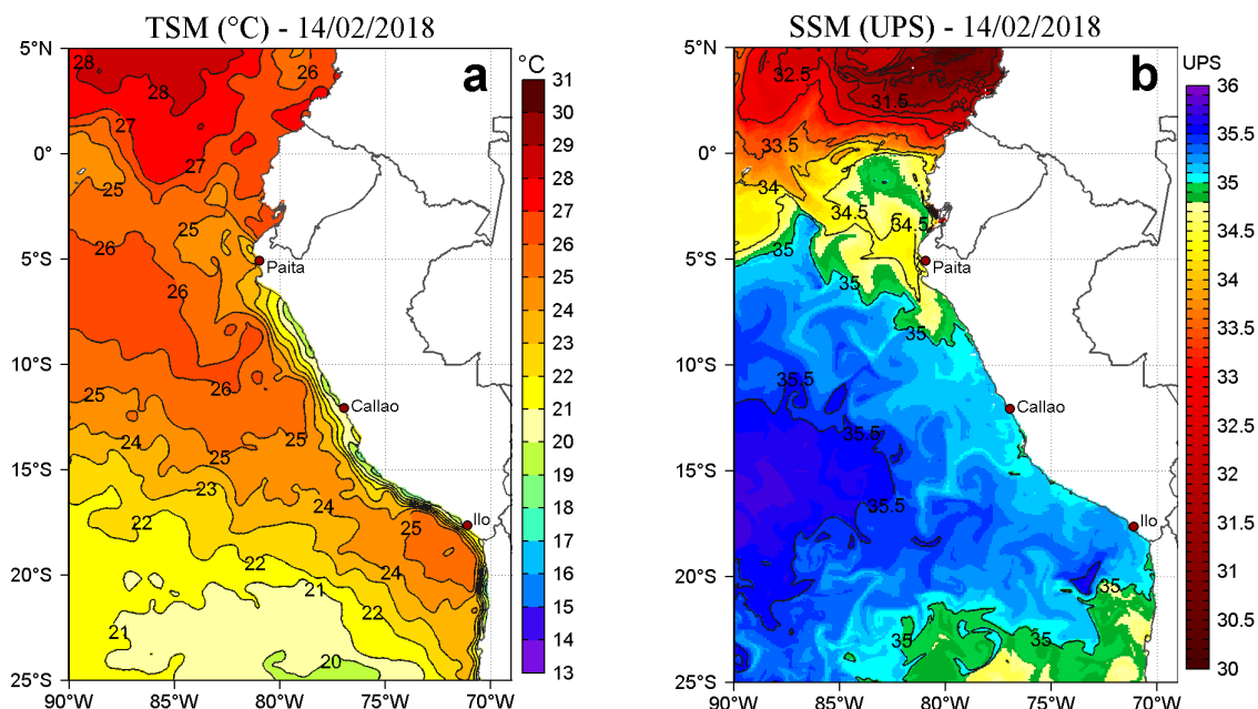
Figura 2. a) Temperatura superficial del mar ( ^{\circ}\text{C} ) y b) Salinidad superficial del mar (UPS) para el 14 de febrero de 2018. Datos: OSTIA-UKMO-L4-GLOB-v2.0 (UK Met Office, 2012; Donlon et al, 2012) disponible en https://podaac.jpl.nasa.gov/dataset/OSTIA-UKMO-L4-GLOB-v2.0 para (a) y Hybrid Coordinate Ocean Model (HYCOM; Halliwell et al., 1998; 2000; Bleck, 2001) para (b). Procesamiento: LHF/AFIOF/DGIOCC/IMARPE.
