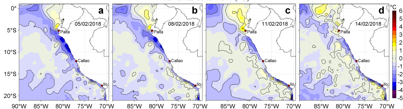
Figura 3. Anomalías de la Temperatura Superficial del Mar ( ^{\circ}\text{C} ) para los días: a) 05, b) 08, c) 11 y d) 14 de febrero de 2018. Las anomalías se calcularon respecto de la climatología para el periodo 2007-2016. Datos: OSTIA-UKMO-L4-GLOB-v2.0 (UK Met Office, 2012; Donlon et al, 2012). Procesamiento: LHF/AFIOF/DGIOCC/IMARPE.
