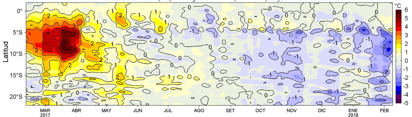
Figura 4. Variación promedio de las anomalías de la Temperatura Superficial del Mar (°C) para una franja de 60 mn (~111 km) adyacente al litoral peruano para los últimos doce meses al 09 de febrero de 2018. Datos: OSTIA-UKMO-L4-GLOB-v2.0 (UK Met. Office, 2012; Donlon et al, 2012) disponible en https://podaac.jpl.nasa.gov/dataset/OSTIA-UKMO-L4-GLOB-v2.0 . Las anomalías se calcularon con respecto al periodo 2007-2016. Procesamiento: LHF/AFIOF/DGIOCC/IMARPE.
