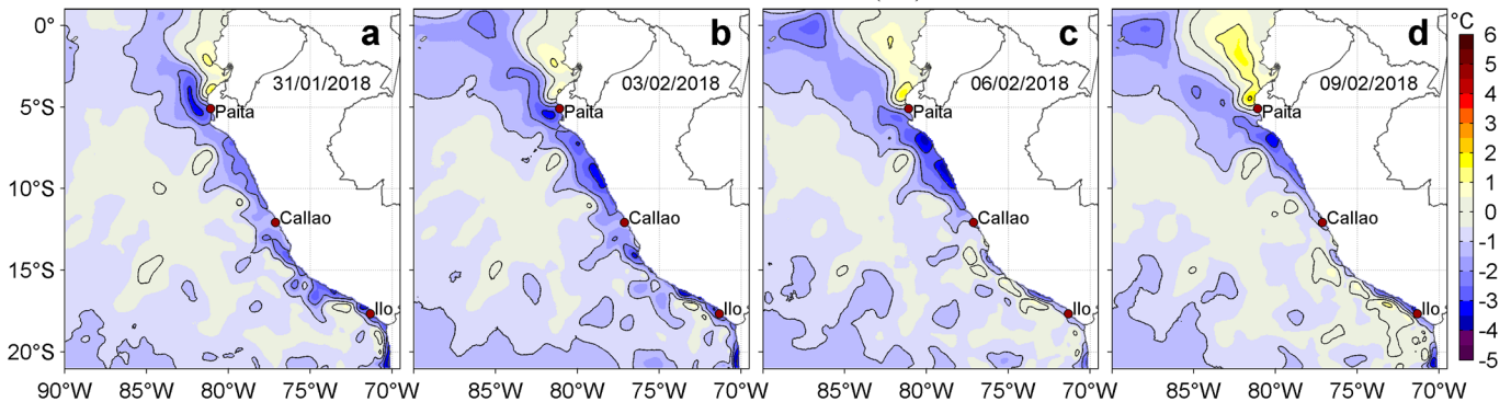
Figura 3. Anomalías de la Temperatura Superficial del Mar (°C) para los días: a) 31 de enero, b) 03, c) 06 y d) 09 de febrero de 2018. Las anomalías se calcularon respecto de la climatología para el periodo 2007-2016. Datos: OSTIA-UKMO-L4-GLOB-v2.0 (UK Met Office, 2012; Donlon et al, 2012). Procesamiento: LHF/AFIOF/DGIOCC/IMARPE.
