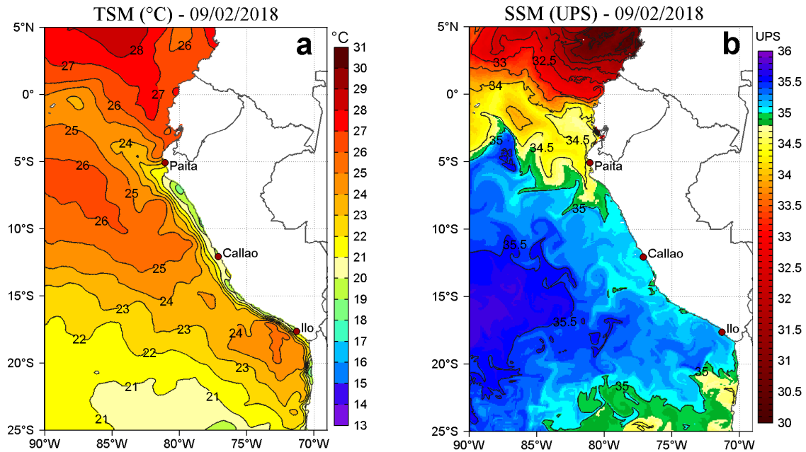
Figura 2. a) Temperatura Superficial del Mar (°C) y b) Salinidad Superficial del Mar (UPS) para el 09 de febrero de 2018. Datos: OSTIA-UKMO-L4-GLOB-v2.0 (UK Met Office, 2012; Donlon et al, 2012) disponible en https://podaac.jpl.nasa.gov/dataset/OSTIA-UKMO-L4-GLOB-v2.0 para (a) y Hybrid Coordinate Ocean Model (HYCOM; Halliwell et al., 1998; 2000; Bleck, 2001) para (b). Procesamiento: LHF/AFIOF/DGIOCC/IMARPE.
