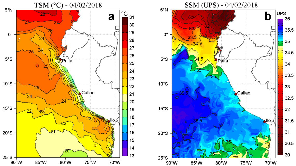
Figura 2. a) Temperatura superficial del mar ( ^{\circ}\text{C} ) y b) Salinidad superficial del mar (UPS) para el 04 de febrero de 2018. Datos: OSTIA-UKMO-L4-GLOB-v2.0 (UK Met Office, 2012; Donlon et al., 2012) disponible en https://podaac.jpl.nasa.gov/dataset/OSTIA-UKMO-L4-GLOB-v2.0 para (a) y Hybrid Coordinate Ocean Model (HYCOM; Halliwell et al., 1998; 2000; Bleck, 2001) para (b). Procesamiento: LHF/AFIOF/DGIOCC/IMARPE.
