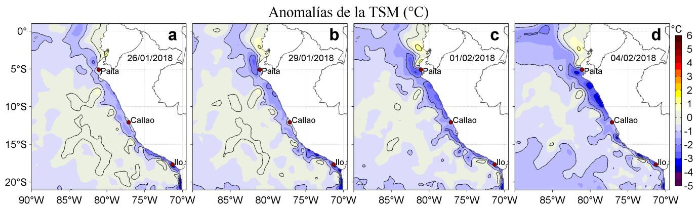
Figura 3. Anomalías de la Temperatura Superficial del Mar ( ^{\circ}\text{C} ) para los días: a) 26, b) 29 de enero, c) 01 y d) 04 de febrero de 2018. Las anomalías se calcularon respecto de la climatología para el periodo 2007-2016. Datos: OSTIA-UKMO-L4-GLOB-v2.0 (UK Met Office, 2012; Donlon et al., 2012). Procesamiento: LHF/AFIOF/DGIOCC/IMARPE.
