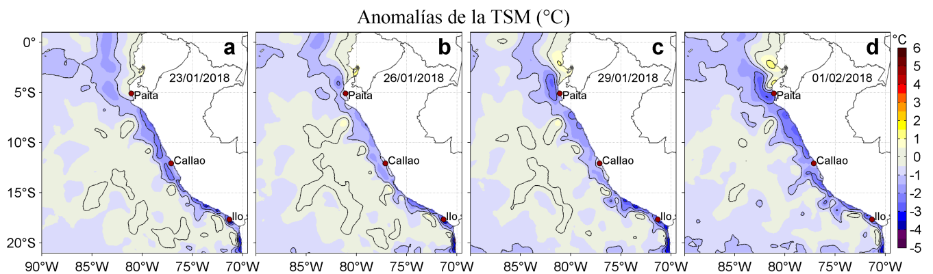
Figura 3. Anomalías de la Temperatura Superficial del Mar ( ^{\circ}\text{C} ) para los días: a) 23, b) 26, c) 29 de enero de 2018 y d) 01 de febrero de 2018. Las anomalías se calcularon respecto de la climatología para el periodo 2007-2016. Datos: OSTIA-UKMO-L4-GLOB-v2.0 (UK Met Office, 2012; Donlon et al, 2012). Procesamiento: LHF/AFIOF/DGIOCC/IMARPE.
