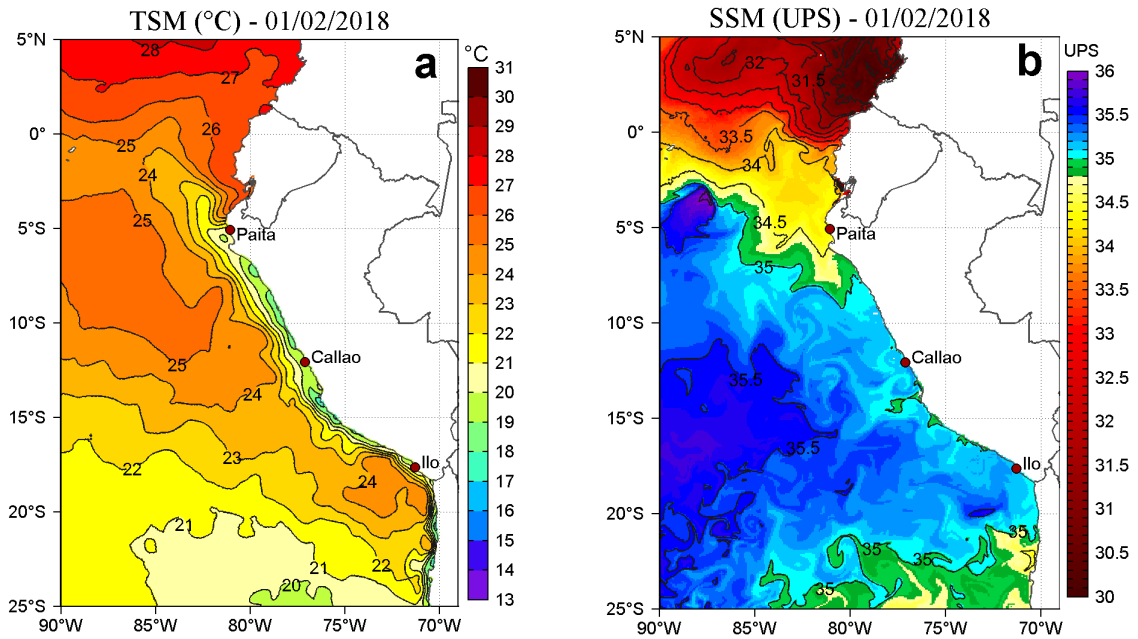
Figura 2. a) Temperatura superficial del mar ( ^{\circ}\text{C} ) y b) Salinidad superficial del mar (UPS) para el 01 de febrero de 2018. Datos: OSTIA-UKMO-L4-GLOB-v2.0 (UK Met Office, 2012; Donlon et al, 2012) disponible en https://podaac.jpl.nasa.gov/dataset/OSTIA-UKMO-L4-GLOB-v2.0 para (a) y Hybrid Coordinate Ocean Model (HYCOM; Halliwell et al., 1998; 2000; Bleck, 2001) para (b). Procesamiento: LHF/AFIOF/DGIOCC/IMARPE.
