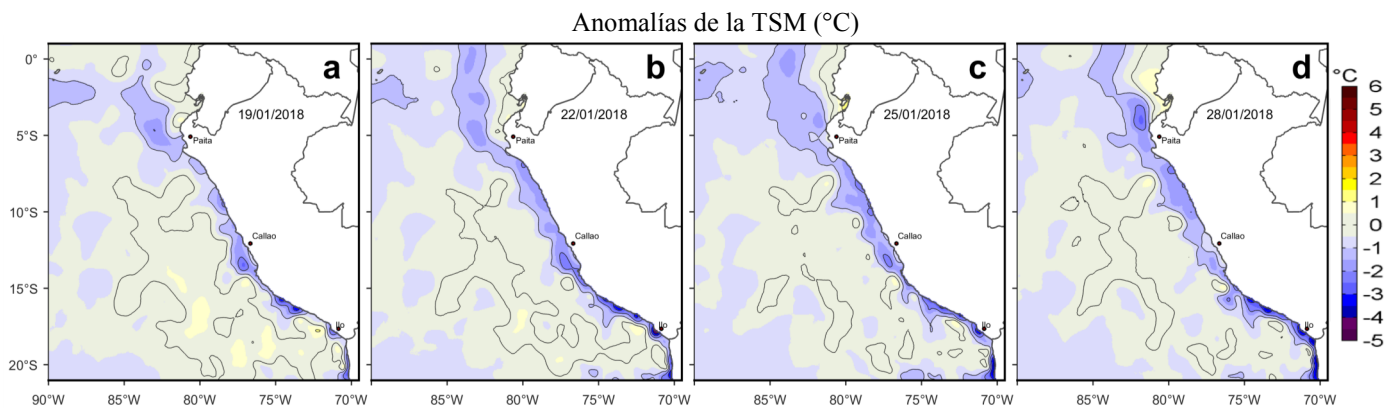
Figura 3. Anomalías de la Temperatura Superficial del Mar (°C) para los días: a) 19, b) 22, c) 25 y d) 28 de enero de 2018. Las anomalías se calcularon respecto de la climatología para el periodo 2007-2016. Datos: OSTIA-UKMO-L4-GLOB-v2.0 (UK Met Office, 2012; Donlon et al, 2012). Procesamiento: LHF/AFIOF/DGIOCC/IMARPE.
