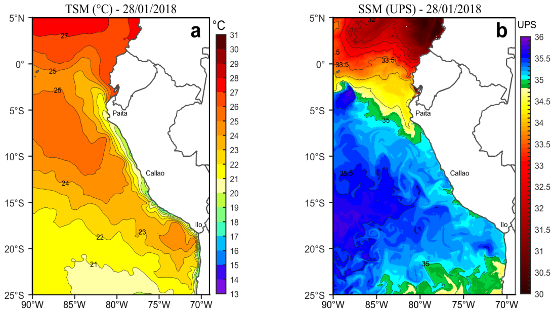
Figura 2. a) Temperatura superficial del mar (°C) y b) Salinidad superficial del mar (UPS) para el 28 de enero de 2018. Datos: OSTIA-UKMO-L4-GLOB-v2.0 (UK Met Office, 2012; Donlon et al, 2012) disponible en https://podaac.jpl.nasa.gov/dataset/OSTIA-UKMO-L4-GLOB-v2.0 para (a) y Hybrid Coordinate Ocean Model (HYCOM; Halliwell et al., 1998; 2000; Bleck, 2001) para (b). Procesamiento: LHF/AFIOF/DGIOCC/IMARPE.
