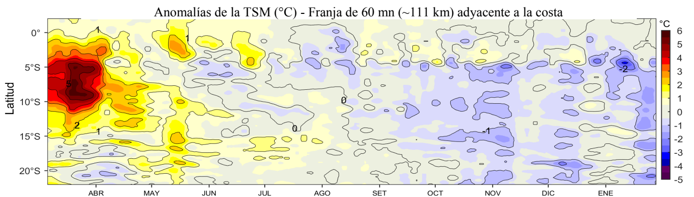
Figura 4. Variación promedio de las anomalías de la Temperatura Superficial del Mar (°C) para una franja de 60 mn (~111 km) adyacente al litoral peruano para los últimos doce meses al 28 de enero de 2018. Datos: OSTIA-UKMO-L4-GLOB-v2.0 (UK Met. Office, 2012; Donlon et al, 2012) disponible en https://podaac.jpl.nasa.gov/dataset/OSTIA-UKMO-L4-GLOB-v2.0 . Las anomalías se calcularon con respecto al periodo 2007-2016. Procesamiento: LHF/AFIOF/DGIOCC/IMARPE.
