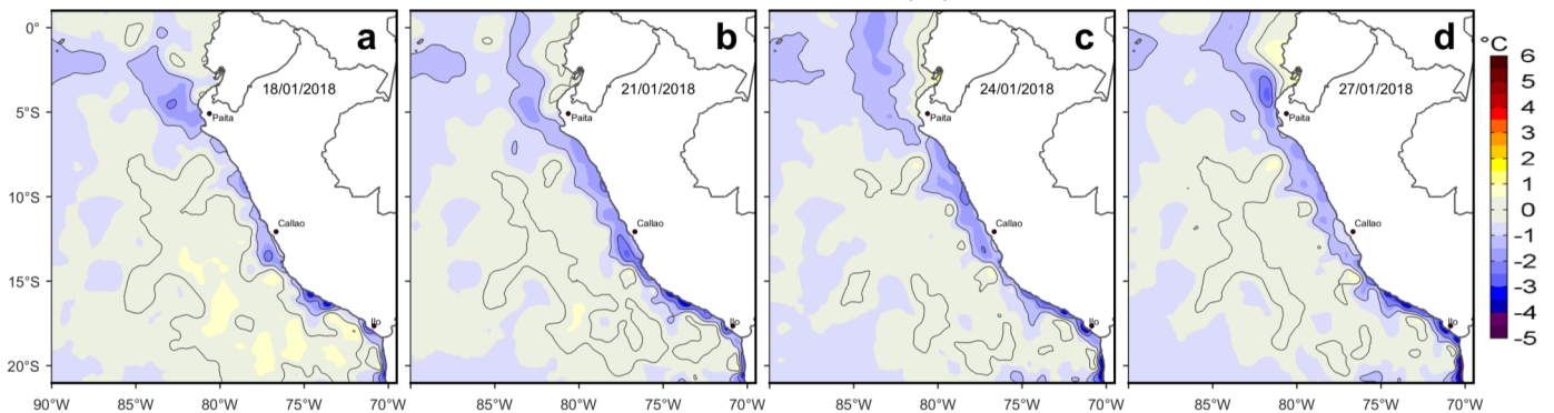
Figura 3. Anomalías de la Temperatura Superficial del Mar ( ^{\circ}\text{C} ) para los días: a) 18, b) 21, c) 24 y d) 27 de enero de 2018. Las anomalías se calcularon respecto de la climatología para el periodo 2007-2016. Datos: OSTIA-UKMO-L4-GLOB-v2.0 (UK Met Office, 2012; Donlon et al, 2012). Procesamiento: LHF/AFIOF/DGIOCC/IMARPE.
