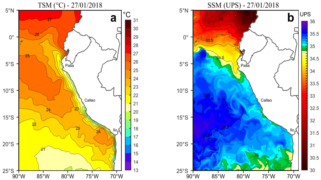
Figura 2. a) Temperatura superficial del mar ( ^{\circ}\text{C} ) y b) Salinidad superficial del mar (UPS) para el 27 de enero de 2018. Datos: OSTIA-UKMO-L4-GLOB-v2.0 (UK Met Office, 2012; Donlon et al, 2012) disponible en https://podaac.jpl.nasa.gov/dataset/OSTIA-UKMO-L4-GLOB-v2.0 para (a) y Hybrid Coordinate Ocean Model (HYCOM; Halliwell et al., 1998; 2000; Bleck, 2001) para (b). Procesamiento: LHF/AFIOF/DGIOCC/IMARPE.
