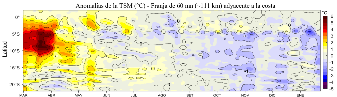
Figura 4. Variación promedio de las anomalías de la Temperatura Superficial del Mar (°C) para una franja de 60 mn (~111 km) adyacente al litoral peruano para los últimos doce meses al 23 de enero de 2018. Datos: OSTIA-UKMO-L4-GLOB-v2.0 (UK Met. Office, 2012; Donlon et al, 2012) disponible en https://podaac.jpl.nasa.gov/dataset/OSTIA-UKMO-L4-GLOB-v2.0 . Las anomalías se calcularon con respecto al periodo 2007-2016. Procesamiento: LHF/AFIOF/DGIOCC/IMARPE.
