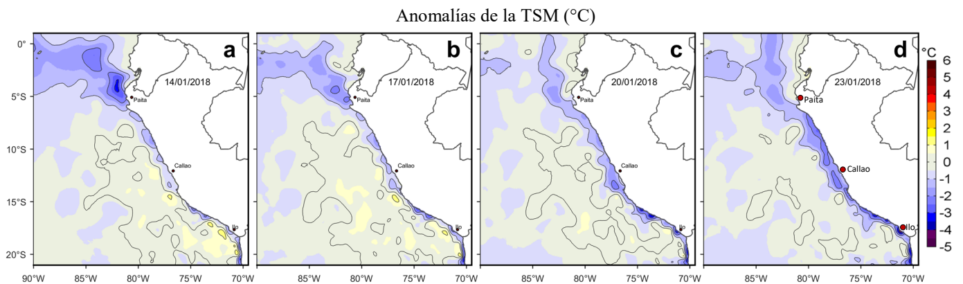
Figura 3. Anomalías de la Temperatura Superficial del Mar (°C) para los días: a) 14, b) 17, c) 20 y d) 23 de enero de 2018. Las anomalías se calcularon respecto de la climatología para el periodo 2007-2016. Datos: OSTIA-UKMO-L4-GLOB-v2.0 (UK Met Office, 2012; Donlon et al, 2012). Procesamiento: LHF/AFIOF/DGIOCC/IMARPE.
