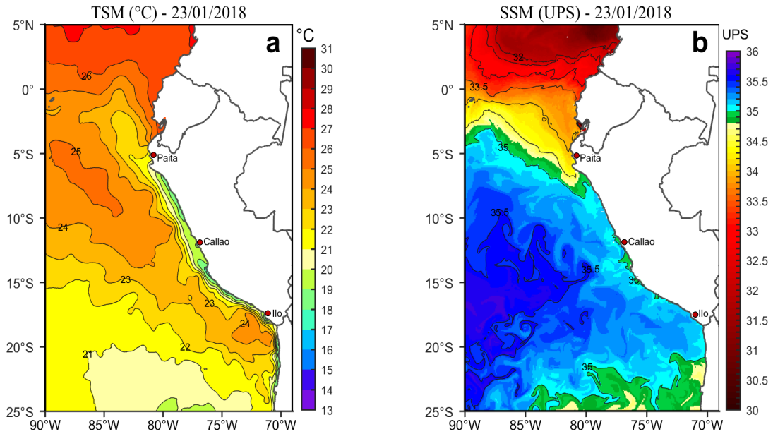
Figura 2. a) Temperatura superficial del mar (°C) y b) Salinidad superficial del mar (UPS) para el 23 de enero de 2018. Datos: OSTIA-UKMO-L4-GLOB-v2.0 (UK Met Office, 2012; Donlon et al, 2012) disponible en https://podaac.jpl.nasa.gov/dataset/OSTIA-UKMO-L4-GLOB-v2.0 para (a) y Hybrid Coordinate Ocean Model (HYCOM; Halliwell et al., 1998; 2000; Bleck, 2001) para (b). Procesamiento: LHF/AFIOF/DGIOCC/IMARPE.
