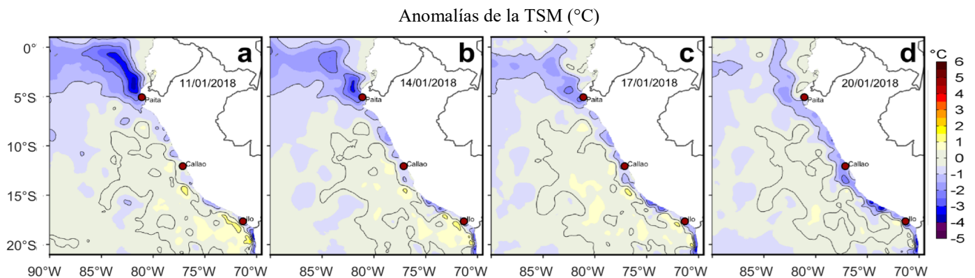
Figura 3. Anomalías de la Temperatura Superficial del Mar ( ^{\circ}\text{C} ) para los días: a) 11, b) 14, c) 17 y d) 20 de enero de 2018. Las anomalías se calcularon respecto de la climatología para el periodo 2007-2016. Datos: OSTIA-UKMO-L4-GLOB-v2.0 (UK Met Office, 2012; Donlon et al, 2012). Procesamiento: LHF/AFIOF/DGIOCC/IMARPE.
