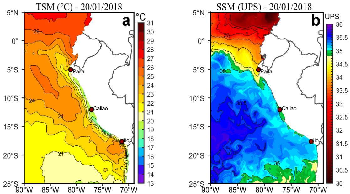
Figura 2. a) Temperatura superficial del mar ( ^{\circ}\text{C} ) y b) Salinidad superficial del mar (UPS) para el 20 de enero de 2018. Datos: OSTIA-UKMO-L4-GLOB-v2.0 (UK Met Office, 2012; Donlon et al, 2012) disponible en https://podaac.jpl.nasa.gov/dataset/OSTIA-UKMO-L4-GLOB-v2.0 para (a) y Hybrid Coordinate Ocean Model (HYCOM; Halliwell et al., 1998; 2000; Bleck, 2001) para (b). Procesamiento: LHF/AFIOF/DGIOCC/IMARPE.
