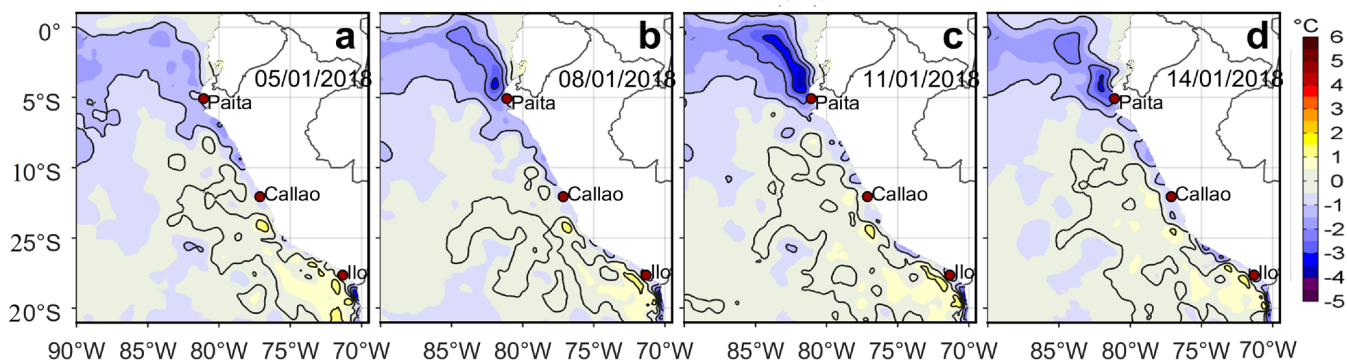
Figura 3. Anomalías de la Temperatura Superficial del Mar ( ^{\circ}\text{C} ) para los días: a) 05, b) 08, c) 11 y d) 14 de enero de 2018. Las anomalías se calcularon respecto de la climatología para el periodo 2007-2016. Datos: OSTIA-UKMO-L4-GLOB-v2.0 (UK Met Office, 2012; Donlon et al, 2012). Procesamiento: LHF/AFIOF/DGIOCC/IMARPE.
