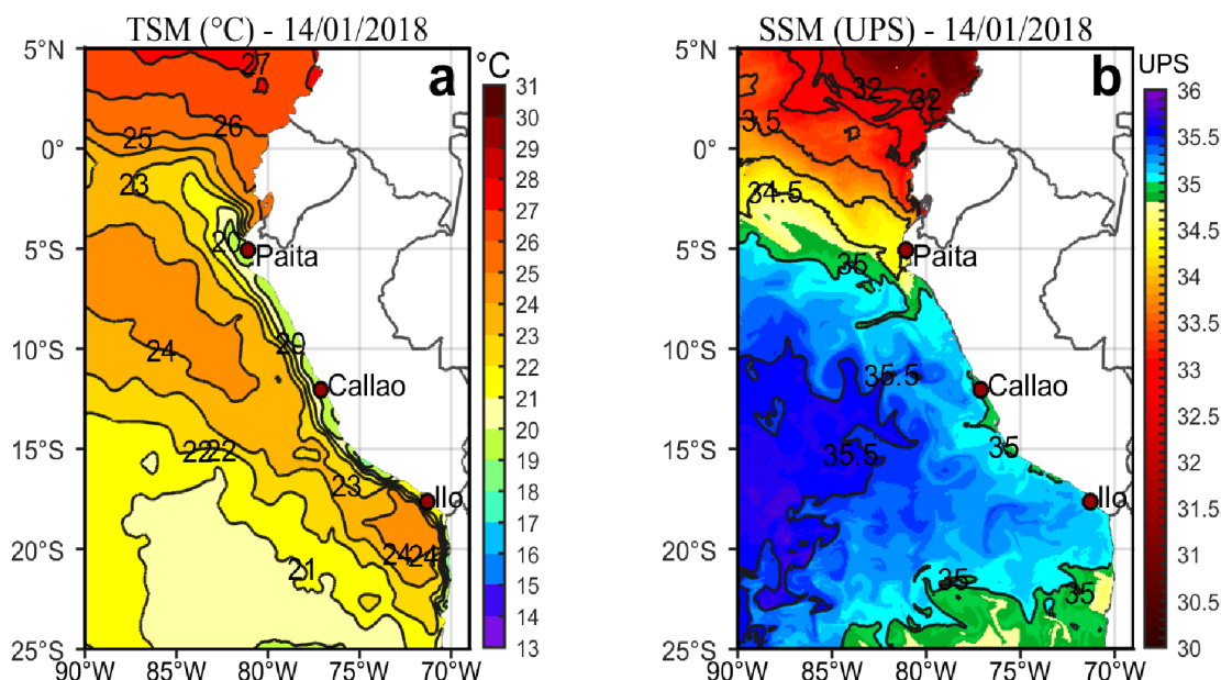
Figura 2. a) Temperatura superficial del mar ( ^{\circ}\text{C} ) y b) Salinidad superficial del mar (UPS) para el 14 de enero de 2018. Datos: OSTIA-UKMO-L4-GLOB-v2.0 (UK Met Office, 2012; Donlon et al, 2012) disponible en https://podaac.jpl.nasa.gov/dataset/OSTIA-UKMO-L4-GLOB-v2.0 para (a) y Hybrid Coordinate Ocean Model (HYCOM; Halliwell et al., 1998; 2000; Bleck, 2001) para (b). Procesamiento: LHF/AFIOF/DGIOCC/IMARPE.
