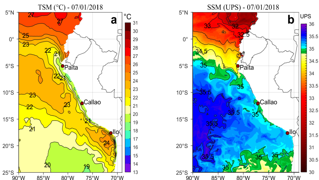
Figura 2. a) Temperatura superficial del mar (°C) y b) Salinidad superficial del mar (UPS) para el 07 de enero. Datos: OSTIA-UKMO-L4-GLOB-v2.0 (UK Met Office, 2012; Donlon et al, 2012) disponible en https://podaac.jpl.nasa.gov/dataset/OSTIA-UKMO-L4-GLOB-v2.0 para (a) y Hybrid Coordinate Ocean Model (HYCOM; Halliwell et al., 1998; 2000; Bleck, 2001) para (b). Procesamiento: LHF/AFIOF/DGIOCC/IMARPE.
