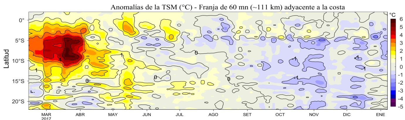
Figura 4. Variación promedio de las anomalías de la temperatura superficial del mar (°C) para una franja de 60 mn (~111 km) adyacente al litoral peruano para los últimos doce meses al 07 de diciembre de 2017. Datos: OSTIA-UKMO-L4-GLOB-v2.0 (UK Met. Office, 2012; Donlon et al, 2012) disponible en https://podaac.jpl.nasa.gov/dataset/OSTIA-UKMO-L4-GLOB-v2.0 . Las anomalías se calcularon con respecto al periodo 2007-2016. Procesamiento: LHF/AFIOF/DGIOCC/IMARPE.
