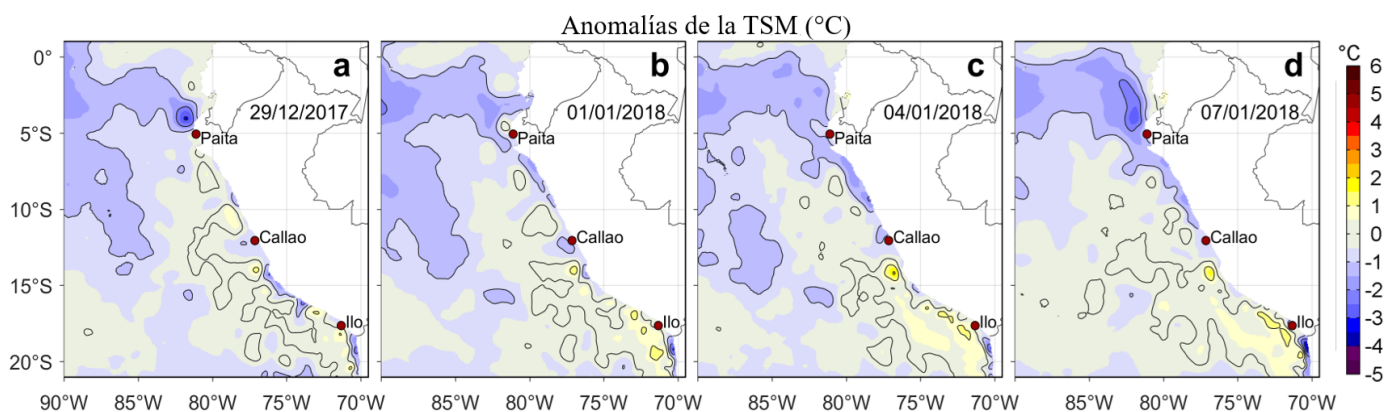
Figura 3. Anomalías de la Temperatura Superficial del Mar (°C) para los días: a) 29 de diciembre de 2017 y b) 01, c) 04 y d) 07 de enero de 2018. Las anomalías se calcularon respecto de la climatología para el periodo 2007-2016. Datos: OSTIA-UKMO-L4-GLOB-v2.0 (UK Met Office, 2012; Donlon et al, 2012). Procesamiento: LHF/AFIOF/DGIOCC/IMARPE.
