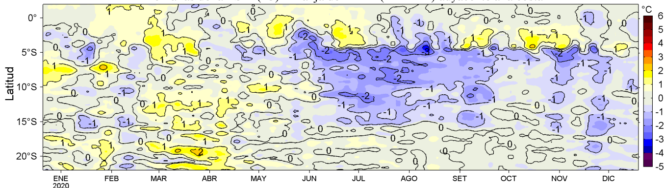
Figura 4. Variación promedio de las anomalías de la temperatura superficial del mar (TSM, °C) para una franja de 60 mn (~111 km) adyacente al litoral peruano para los últimos doce meses al 19 de diciembre de 2020. Datos: OSTIA-UKMO-L4-GLOB-v2.0 (UK Met. Office, 2012; Donlon et al, 2012) disponible en https://podaac.jpl.nasa.gov/dataset/OSTIA-UKMO-L4-GLOB-v2.0 . Las anomalías se calcularon con respecto al periodo 2007-2016. Procesamiento: LHFMAFIOF/DGIOCC.
