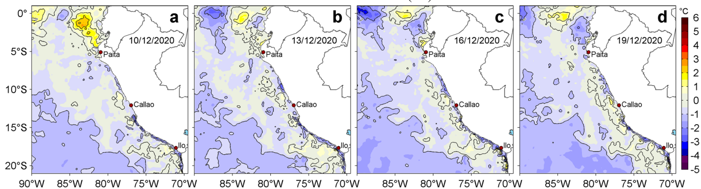
Figura 3. Anomalías de la temperatura superficial del mar (TSM, °C) para los días: a) 10, b) 13, c) 16 y d) 19 de diciembre de 2020. Las anomalías se calcularon respecto de la climatología para el periodo 2007-2016. Datos: OSTIA-UKMO-L4-GLOB-v2.0 (UK Met Office, 2012; Donlon et al, 2012). Procesamiento: LHFMAFIOF/DGIOCC.
