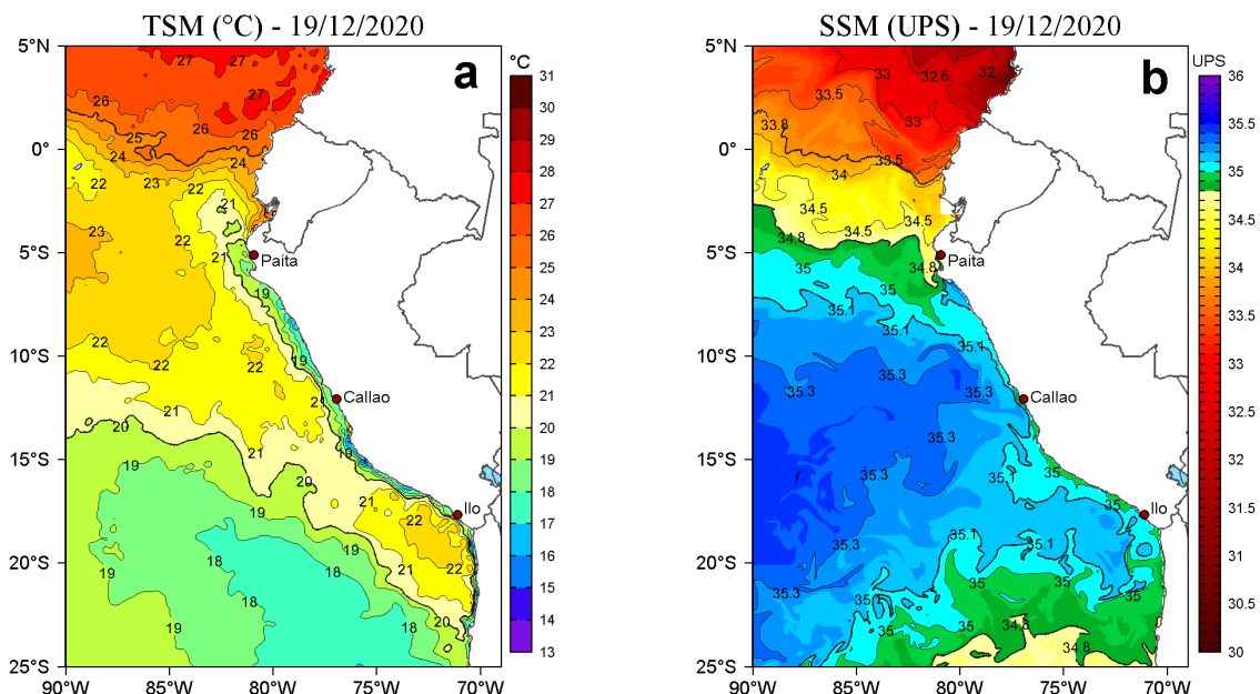
Figura 2. a) Temperatura superficial del mar (TSM, °C) y b) Salinidad superficial del mar (SSM, UPS), para el 19 de diciembre de 2020. Datos: OSTIA-UKMO-L4-GLOB-v2.0 (UK Met Office, 2012; Donlon et al, 2012) disponible en https://podaac.jpl.nasa.gov/dataset/OSTIA-UKMO-L4-GLOB-v2.0 para (a) y Hybrid Coordinate Ocean Model v. GOFS 3.1 (HYCOM; Halliwell et al., 1998; 2000; Bleck, 2001) para (b). Procesamiento: LHFMAFIOF/DGIOCC.
