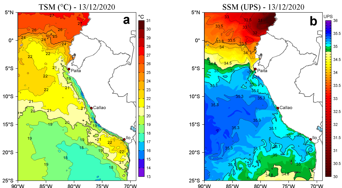
Figura 2. a) Temperatura superficial del mar (TSM, °C) y b) Salinidad superficial del mar (SSM, UPS), para el 13 de diciembre de 2020. Datos: OSTIA-UKMO-L4-GLOB-v2.0 (UK Met Office, 2012; Donlon et al, 2012) disponible en https://podaac.jpl.nasa.gov/dataset/OSTIA-UKMO-L4-GLOB-v2.0 para (a) y Hybrid Coordinate Ocean Model v. GOFS 3.1 (HYCOM; Halliwell et al., 1998; 2000; Bleck, 2001) para (b). Procesamiento: LHFMAFIOF/DGIOCC.
