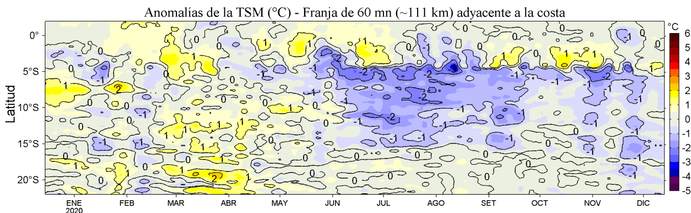
Figura 4. Variación promedio de las anomalías de la temperatura superficial del mar (TSM, °C) para una franja de 60 mn (~111 km) adyacente al litoral peruano para los últimos doce meses al 13 de diciembre de 2020. Datos: OSTIA-UKMO-L4-GLOB-v2.0 (UK Met. Office, 2012; Donlon et al, 2012) disponible en https://podaac.jpl.nasa.gov/dataset/OSTIA-UKMO-L4-GLOB-v2.0 . Las anomalías se calcularon con respecto al periodo 2007-2016. Procesamiento: LHFMAFIOF/DGIOCC.
