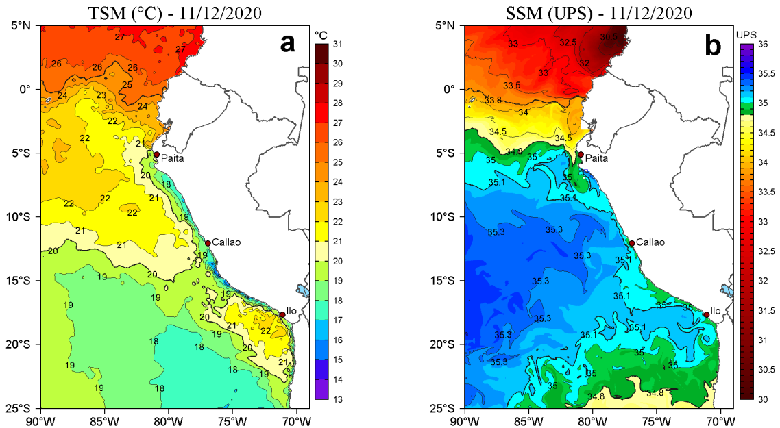
Figura 2. a) Temperatura superficial del mar (TSM, °C) y b) Salinidad superficial del mar (SSM, UPS), para el 11 de diciembre de 2020. Datos: OSTIA-UKMO-L4-GLOB-v2.0 (UK Met Office, 2012; Donlon et al, 2012) disponible en https://podaac.jpl.nasa.gov/dataset/OSTIA-UKMO-L4-GLOB-v2.0 para (a) y Hybrid Coordinate Ocean Model v. GOFS 3.1 (HYCOM; Halliwell et al., 1998; 2000; Bleck, 2001) para (b). Procesamiento: LHFMAFIOF/DGIOCC.
