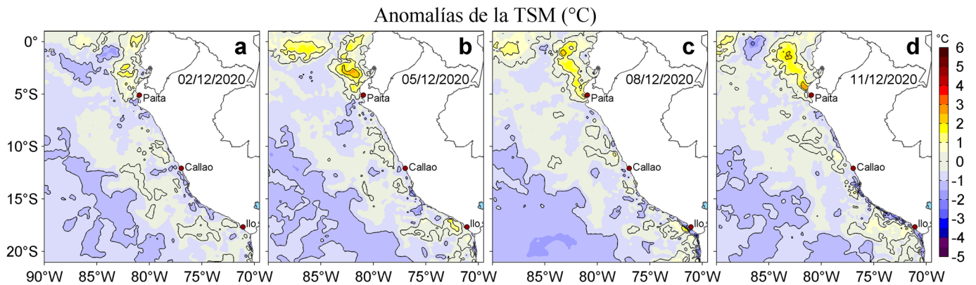
Figura 3. Anomalías de la temperatura superficial del mar (TSM, °C) para los días: a) 02, b) 05, c) 08 y d) 11 de diciembre de 2020. Las anomalías se calcularon respecto de la climatología para el periodo 2007-2016. Datos: OSTIA-UKMO-L4-GLOB-v2.0 (UK Met Office, 2012; Donlon et al, 2012). Procesamiento: LHFMAFIOF/DGIOCC.
