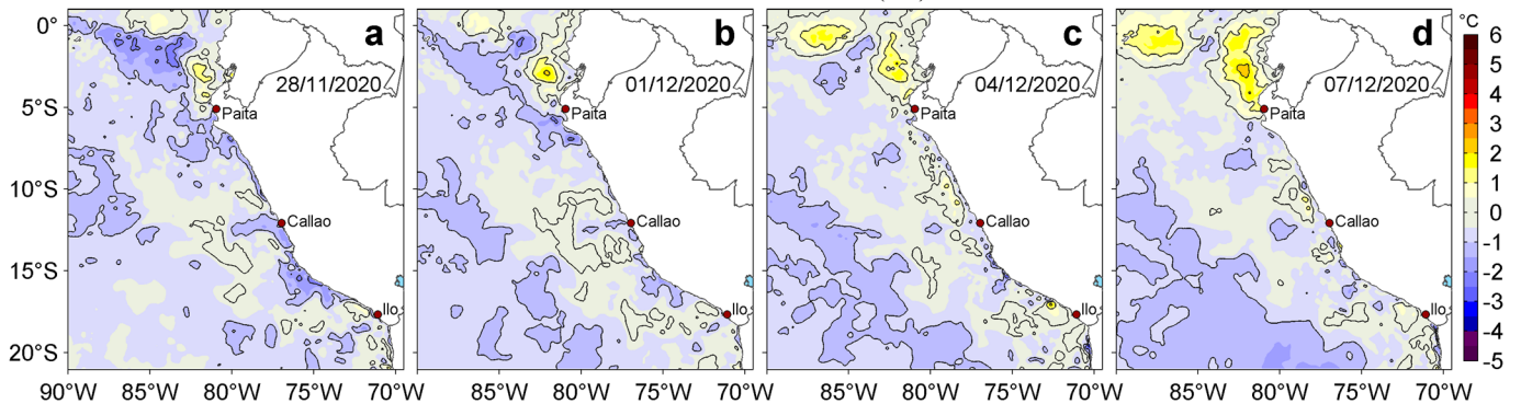
Figura 3. Anomalías de la temperatura superficial del mar (TSM, °C) para los días: a) 28 de noviembre, b) 01, c) 04 y d) 07 de diciembre de 2020. Las anomalías se calcularon respecto de la climatología para el periodo 2007-2016. Datos: OSTIA-UKMO-L4-GLOB-v2.0 (UK Met Office, 2012; Donlon et al, 2012). Procesamiento: LHFMAFIOF/DGIOCC.
