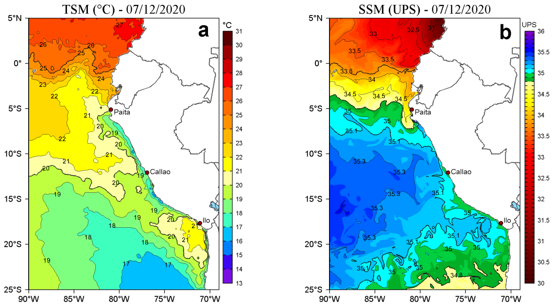
Figura 2. a) Temperatura superficial del mar (TSM, °C) y b) Salinidad superficial del mar (SSM, UPS), para el 07 de diciembre de 2020. Datos: OSTIA-UKMO-L4-GLOB-v2.0 (UK Met Office, 2012; Donlon et al, 2012) disponible en https://podaac.jpl.nasa.gov/dataset/OSTIA-UKMO-L4-GLOB-v2.0 para (a) y Hybrid Coordinate Ocean Model v. GOFS 3.1 (HYCOM; Halliwell et al., 1998; 2000; Bleck, 2001) para (b). Procesamiento: LHFMAFIOF/DGIOCC.
