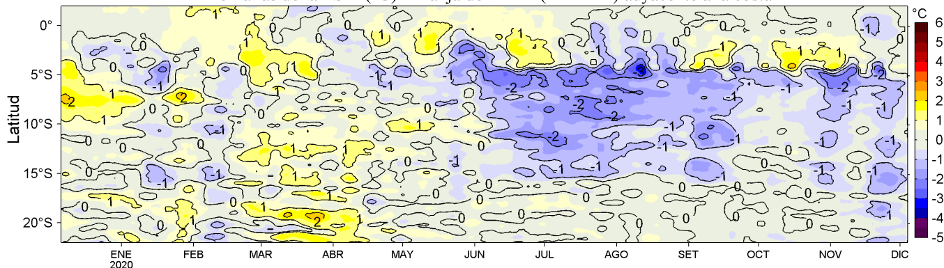
Figura 4. Variación promedio de las anomalías de la temperatura superficial del mar (TSM, °C) para una franja de 60 mn (~111 km) adyacente al litoral peruano para los últimos doce meses al 04 de diciembre de 2020. Datos: OSTIA-UKMO-L4-GLOB-v2.0 (UK Met. Office, 2012; Donlon et al, 2012) disponible en https://podaac.jpl.nasa.gov/dataset/OSTIA-UKMO-L4-GLOB-v2.0 . Las anomalías se calcularon con respecto al periodo 2007-2016. Procesamiento: LHFm/AFIOF/DGIOCC.
