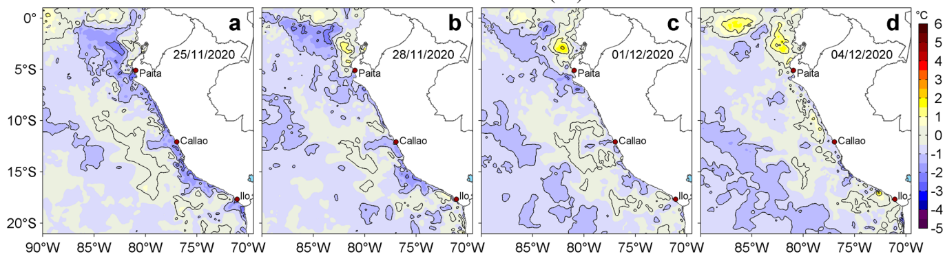
Figura 3. Anomalías de la temperatura superficial del mar (TSM, °C) para los días: a) 25 y b) 28 de noviembre, c) 01 y d) 04 de diciembre de 2020. Las anomalías se calcularon respecto de la climatología para el periodo 2007-2016. Datos: OSTIA-UKMO-L4-GLOB-v2.0 (UK Met Office, 2012; Donlon et al, 2012). Procesamiento: LHFm/AFIOF/DGIOCC.
