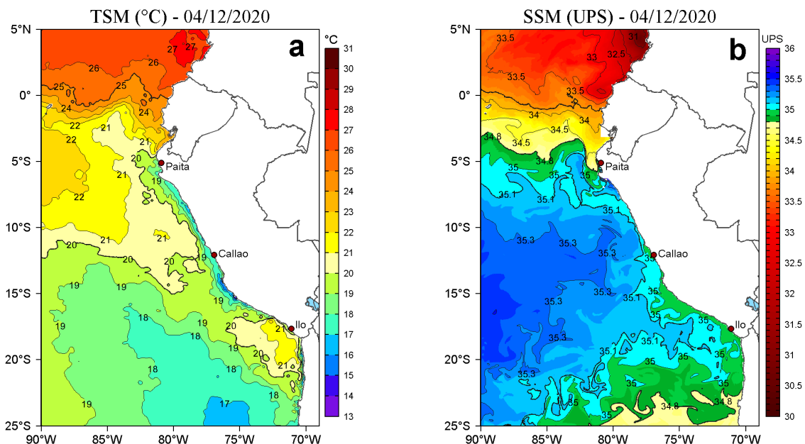
Figura 2. a) Temperatura superficial del mar (TSM, °C) y b) Salinidad superficial del mar (SSM, UPS), para el 04 de diciembre de 2020. Datos: OSTIA-UKMO-L4-GLOB-v2.0 (UK Met Office, 2012; Donlon et al, 2012) disponible en https://podaac.jpl.nasa.gov/dataset/OSTIA-UKMO-L4-GLOB-v2.0 para (a) y Hybrid Coordinate Ocean Model v. GOFS 3.1 (HYCOM; Halliwell et al., 1998; 2000; Bleck, 2001) para (b). Procesamiento: LHFm/AFIOF/DGIOCC.
