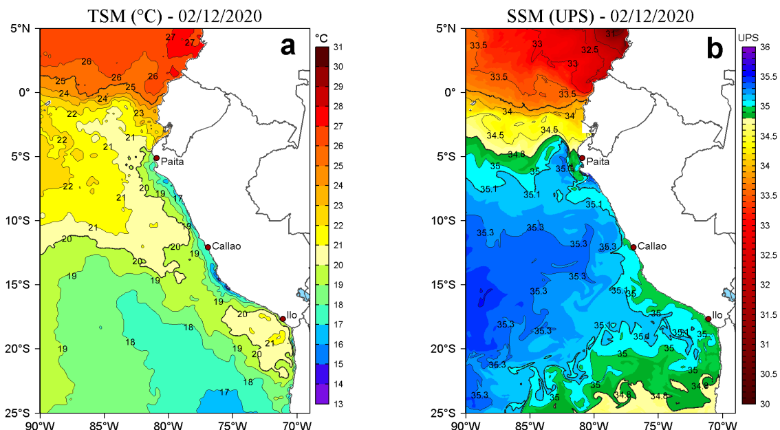
Figura 2. a) Temperatura superficial del mar (TSM, °C) y b) Salinidad superficial del mar (SSM, UPS), para el 02 de diciembre de 2020. Datos: OSTIA-UKMO-L4-GLOB-v2.0 (UK Met Office, 2012; Donlon et al, 2012) disponible en https://podaac.jpl.nasa.gov/dataset/OSTIA-UKMO-L4-GLOB-v2.0 para (a) y Hybrid Coordinate Ocean Model v. GOFS 3.1 (HYCOM; Halliwell et al., 1998; 2000; Bleck, 2001) para (b). Procesamiento: LHF/AFIOF/DGIOCC.
