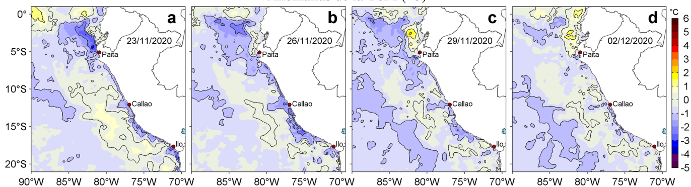
Figura 3. Anomalías de la temperatura superficial del mar (TSM, °C) para los días: a) 23, b) 26 y c) 29 de noviembre y d) 02 de diciembre de 2020. Las anomalías se calcularon respecto de la climatología para el periodo 2007-2016. Datos: OSTIA-UKMO-L4-GLOB-v2.0 (UK Met Office, 2012; Donlon et al, 2012). Procesamiento: LHF/AFIOF/DGIOCC.
