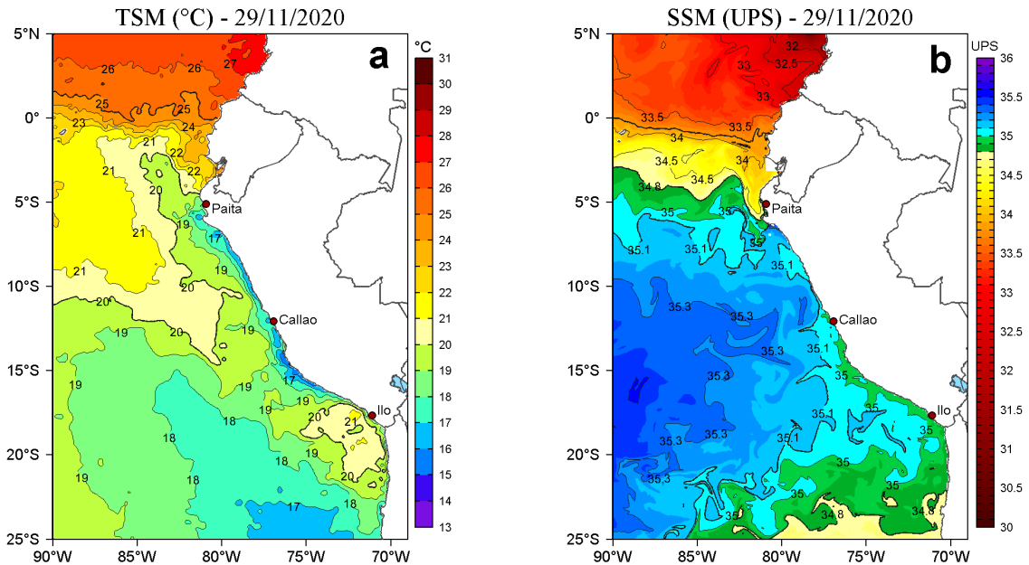
Figura 2. a) Temperatura superficial del mar (TSM, °C) y b) Salinidad superficial del mar (SSM, UPS), para el 29 de noviembre de 2020. Datos: OSTIA-UKMO-L4-GLOB-v2.0 (UK Met Office, 2012; Donlon et al, 2012) disponible en https://podaac.jpl.nasa.gov/dataset/OSTIA-UKMO-L4-GLOB-v2.0 para (a) y Hybrid Coordinate Ocean Model v. GOFS 3.1 (HYCOM; Halliwell et al., 1998; 2000; Bleck, 2001) para (b). Procesamiento: LHFV/AFIOF/DGIOCC.
