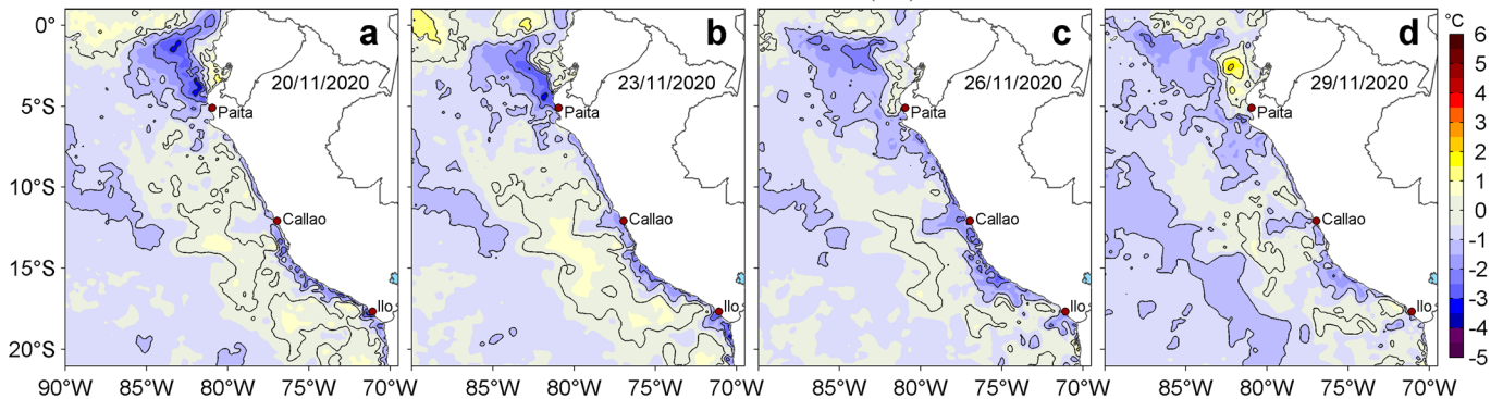
Figura 3. Anomalías de la temperatura superficial del mar (TSM, °C) para los días: a) 20, b) 23, c) 26 y d) 29 de noviembre de 2020. Las anomalías se calcularon respecto de la climatología para el periodo 2007-2016. Datos: OSTIA-UKMO-L4-GLOB-v2.0 (UK Met Office, 2012; Donlon et al, 2012). Procesamiento: LHFV/AFIOF/DGIOCC.
