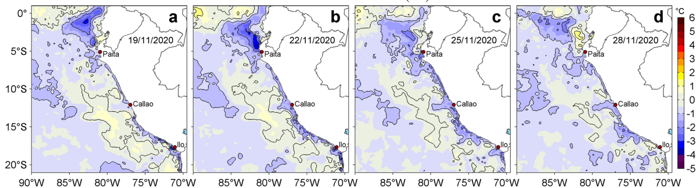
Figura 3. Anomalías de la temperatura superficial del mar (TSM, °C) para los días: a) 19, b) 22, c) 25 y d) 28 de noviembre de 2020. Las anomalías se calcularon respecto de la climatología para el periodo 2007-2016. Datos: OSTIA-UKMO-L4-GLOB-v2.0 (UK Met Office, 2012; Donlon et al, 2012). Procesamiento: LHFMAFIOF/DGIOCC.
