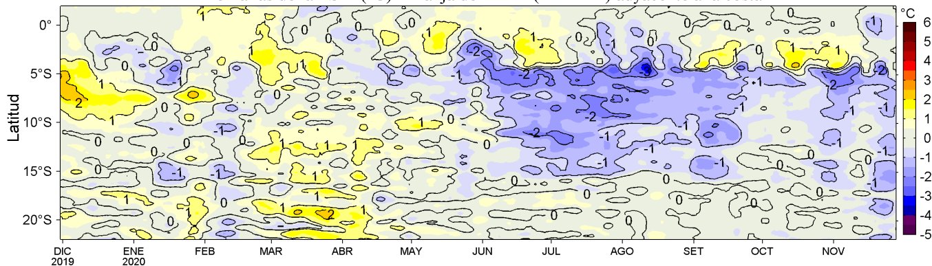
Figura 4. Variación promedio de las anomalías de la temperatura superficial del mar (TSM, °C) para una franja de 60 mn (~111 km) adyacente al litoral peruano para los últimos doce meses al 28 de noviembre de 2020. Datos: OSTIA-UKMO-L4-GLOB-v2.0 (UK Met. Office, 2012; Donlon et al, 2012) disponible en https://podaac.jpl.nasa.gov/dataset/OSTIA-UKMO-L4-GLOB-v2.0 . Las anomalías se calcularon con respecto al periodo 2007-2016. Procesamiento: LHFMAFIOF/DGIOCC.
