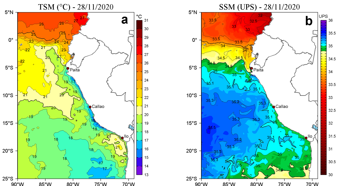
Figura 2. a) Temperatura superficial del mar (TSM, °C) y b) Salinidad superficial del mar (SSM, UPS), para el 28 de noviembre de 2020. Datos: OSTIA-UKMO-L4-GLOB-v2.0 (UK Met Office, 2012; Donlon et al, 2012) disponible en https://podaac.jpl.nasa.gov/dataset/OSTIA-UKMO-L4-GLOB-v2.0 para (a) y Hybrid Coordinate Ocean Model v. GOFS 3.1 (HYCOM; Halliwell et al., 1998; 2000; Bleck, 2001) para (b). Procesamiento: LHFMAFIOF/DGIOCC.
