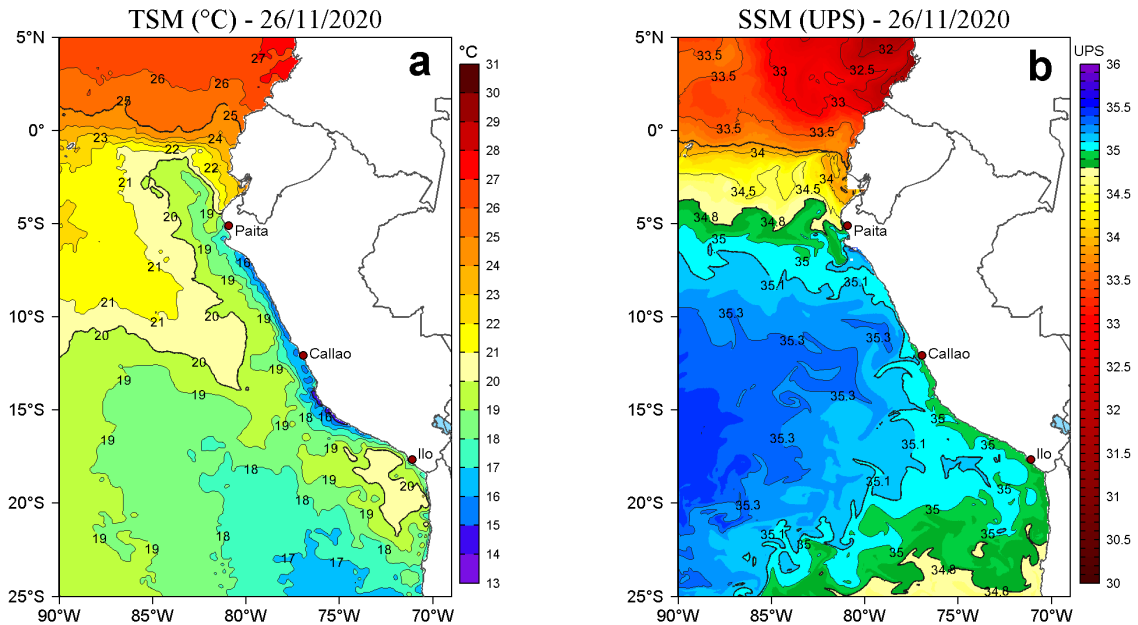
Figura 2. a) Temperatura superficial del mar (TSM, °C) y b) Salinidad superficial del mar (SSM, UPS), para el 26 de noviembre de 2020. Datos: OSTIA-UKMO-L4-GLOB-v2.0 (UK Met Office, 2012; Donlon et al, 2012) disponible en https://podaac.jpl.nasa.gov/dataset/OSTIA-UKMO-L4-GLOB-v2.0 para (a) y Hybrid Coordinate Ocean Model v. GOFS 3.1 (HYCOM; Halliwell et al., 1998; 2000; Bleck, 2001) para (b). Procesamiento: LHFMAFIOF/DGIOCC.
