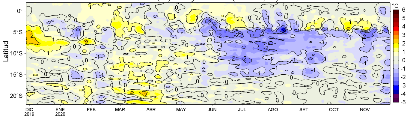
Figura 4. Variación promedio de las anomalías de la temperatura superficial del mar (TSM, °C) para una franja de 60 mn (~111 km) adyacente al litoral peruano para los últimos doce meses al 26 de noviembre de 2020. Datos: OSTIA-UKMO-L4-GLOB-v2.0 (UK Met. Office, 2012; Donlon et al, 2012) disponible en https://podaac.jpl.nasa.gov/dataset/OSTIA-UKMO-L4-GLOB-v2.0 . Las anomalías se calcularon con respecto al periodo 2007-2016. Procesamiento: LHFMAFIOF/DGIOCC.
