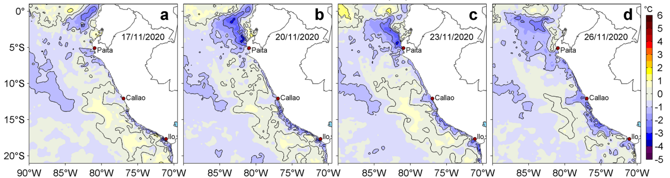
Figura 3. Anomalías de la temperatura superficial del mar (TSM, °C) para los días: a) 17, b) 20, c) 23 y d) 26 de noviembre de 2020. Las anomalías se calcularon respecto de la climatología para el periodo 2007-2016. Datos: OSTIA-UKMO-L4-GLOB-v2.0 (UK Met Office, 2012; Donlon et al, 2012). Procesamiento: LHFMAFIOF/DGIOCC.
