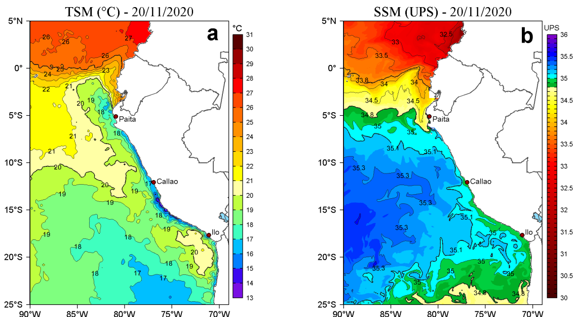
Figura 2. a) Temperatura superficial del mar (TSM, °C) y b) Salinidad superficial del mar (SSM, UPS), para el 20 de noviembre de 2020. Datos: OSTIA-UKMO-L4-GLOB-v2.0 (UK Met Office, 2012; Donlon et al, 2012) disponible en https://podaac.jpl.nasa.gov/dataset/OSTIA-UKMO-L4-GLOB-v2.0 para (a) y Hybrid Coordinate Ocean Model v. GOFS 3.1 (HYCOM; Halliwell et al., 1998; 2000; Bleck, 2001) para (b). Procesamiento: LHF/AFIOF/DGIOCC.
