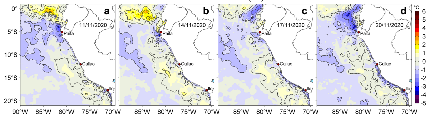
Figura 3. Anomalías de la temperatura superficial del mar (TSM, °C) para los días: a) 11, b) 14, c) 17 y d) 20 de noviembre de 2020. Las anomalías se calcularon respecto de la climatología para el periodo 2007-2016. Datos: OSTIA-UKMO-L4-GLOB-v2.0 (UK Met Office, 2012; Donlon et al, 2012). Procesamiento: LHF/AFIOF/DGIOCC.
