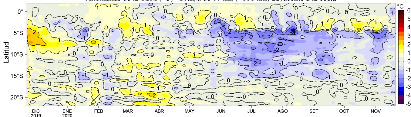
Figura 4. Variación promedio de las anomalías de la temperatura superficial del mar (TSM, °C) para una franja de 60 mn (~111 km) adyacente al litoral peruano para los últimos doce meses al 20 de noviembre de 2020. Datos: OSTIA-UKMO-L4-GLOB-v2.0 (UK Met. Office, 2012; Donlon et al, 2012) disponible en https://podaac.jpl.nasa.gov/dataset/OSTIA-UKMO-L4-GLOB-v2.0 . Las anomalías se calcularon con respecto al periodo 2007-2016. Procesamiento: LHF/AFIOF/DGIOCC.
