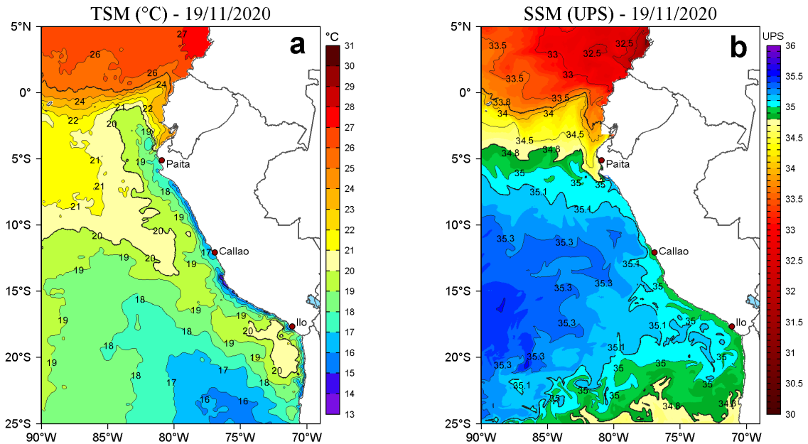
Figura 2. a) Temperatura superficial del mar (TSM, °C) y b) Salinidad superficial del mar (SSM, UPS), para el 19 de noviembre de 2020. Datos: OSTIA-UKMO-L4-GLOB-v2.0 (UK Met Office, 2012; Donlon et al, 2012) disponible en https://podaac.jpl.nasa.gov/dataset/OSTIA-UKMO-L4-GLOB-v2.0 para (a) y Hybrid Coordinate Ocean Model v. GOFS 3.1 (HYCOM; Halliwell et al., 1998; 2000; Bleck, 2001) para (b). Procesamiento: LHFMAFIOF/DGIOCC.
