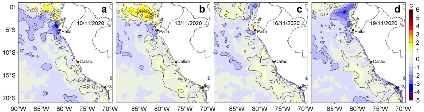
Figura 3. Anomalías de la temperatura superficial del mar (TSM, °C) para los días: a) 10, b) 13, c) 16 y d) 19 de noviembre de 2020. Las anomalías se calcularon respecto de la climatología para el periodo 2007-2016. Datos: OSTIA-UKMO-L4-GLOB-v2.0 (UK Met Office, 2012; Donlon et al, 2012). Procesamiento: LHFMAFIOF/DGIOCC.
