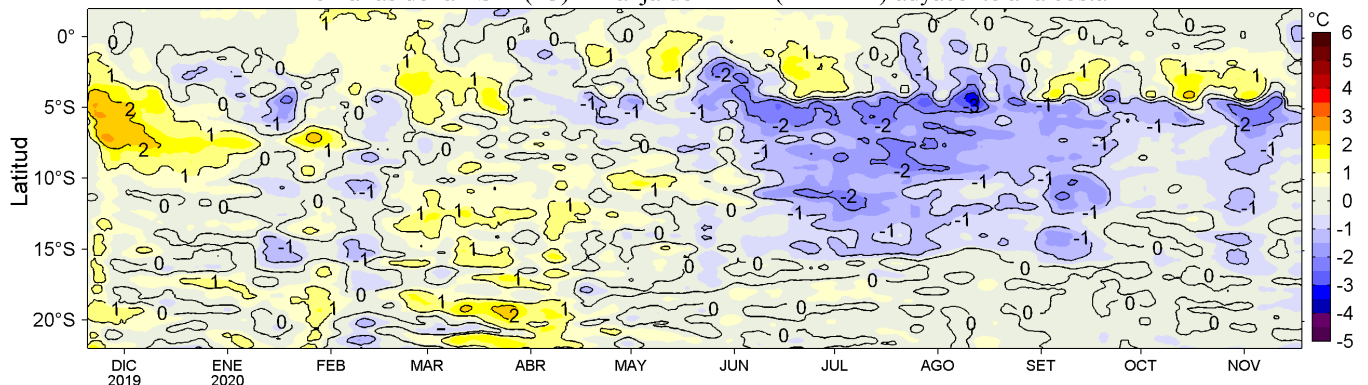
Figura 4. Variación promedio de las anomalías de la temperatura superficial del mar (TSM, °C) para una franja de 60 mn (~111 km) adyacente al litoral peruano para los últimos doce meses al 18 de noviembre de 2020. Datos: OSTIA-UKMO-L4-GLOB-v2.0 (UK Met. Office, 2012; Donlon et al, 2012) disponible en https://podaac.jpl.nasa.gov/dataset/OSTIA-UKMO-L4-GLOB-v2.0 . Las anomalías se calcularon con respecto al periodo 2007-2016. Procesamiento: LHF/AFIOF/DGIOCC.
