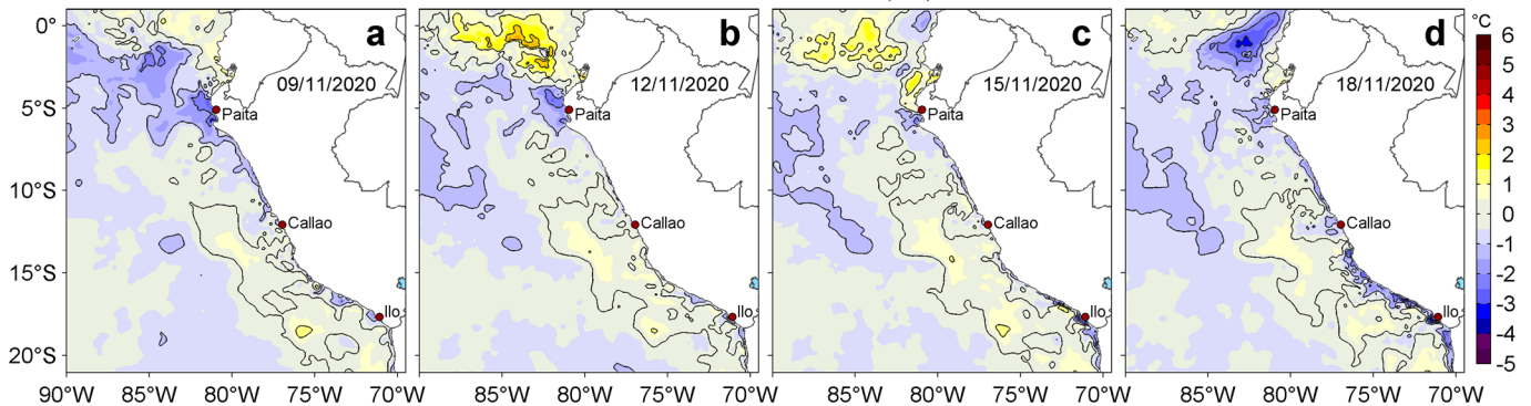
Figura 3. Anomalías de la temperatura superficial del mar (TSM, °C) para los días: a) 09, b) 12, c) 15 y d) 18 de noviembre de 2020. Las anomalías se calcularon respecto de la climatología para el periodo 2007-2016. Datos: OSTIA-UKMO-L4-GLOB-v2.0 (UK Met Office, 2012; Donlon et al, 2012). Procesamiento: LHF/AFIOF/DGIOCC.
