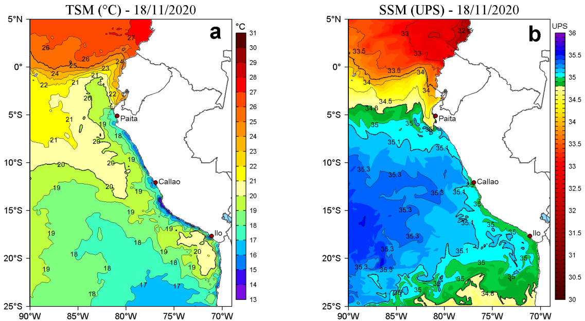
Figura 2. a) Temperatura superficial del mar (TSM, °C) y b) Salinidad superficial del mar (SSM, UPS), para el 18 de noviembre de 2020. Datos: OSTIA-UKMO-L4-GLOB-v2.0 (UK Met Office, 2012; Donlon et al, 2012) disponible en https://podaac.jpl.nasa.gov/dataset/OSTIA-UKMO-L4-GLOB-v2.0 para (a) y Hybrid Coordinate Ocean Model v. GOFS 3.1 (HYCOM; Halliwell et al., 1998; 2000; Bleck, 2001) para (b). Procesamiento: LHF/AFIOF/DGIOCC.
