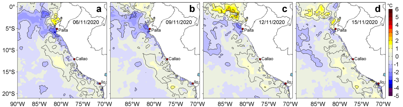
Figura 3. Anomalías de la temperatura superficial del mar (TSM, °C) para los días: a) 06, b) 09, c) 12 y d) 15 de noviembre de 2020. Las anomalías se calcularon respecto de la climatología para el periodo 2007-2016. Datos: OSTIA-UKMO-L4-GLOB-v2.0 (UK Met Office, 2012; Donlon et al, 2012). Procesamiento: LHF/AFIOF/DGIOCC.
