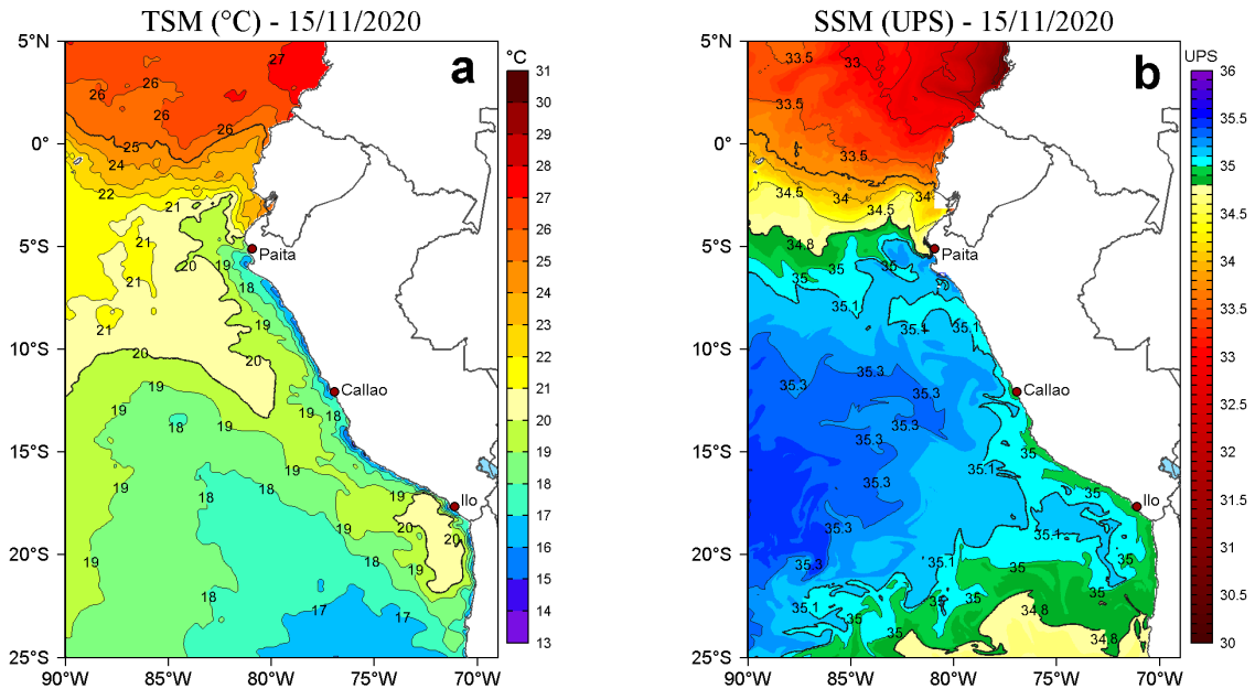
Figura 2. a) Temperatura superficial del mar (TSM, °C) y b) Salinidad superficial del mar (SSM, UPS), para el 15 de noviembre de 2020. Datos: OSTIA-UKMO-L4-GLOB-v2.0 (UK Met Office, 2012; Donlon et al, 2012) disponible en https://podaac.jpl.nasa.gov/dataset/OSTIA-UKMO-L4-GLOB-v2.0 para (a) y Hybrid Coordinate Ocean Model v. GOFS 3.1 (HYCOM; Halliwell et al., 1998; 2000; Bleck, 2001) para (b). Procesamiento: LHF/AFIOF/DGIOCC.
