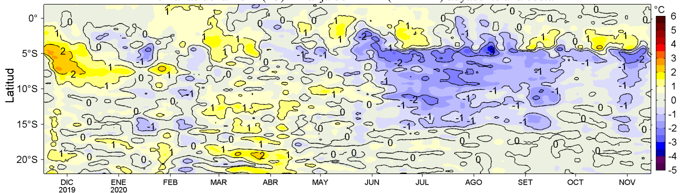
Figura 4. Variación promedio de las anomalías de la temperatura superficial del mar (TSM, °C) para una franja de 60 mn (~111 km) adyacente al litoral peruano para los últimos doce meses al 15 de noviembre de 2020. Datos: OSTIA-UKMO-L4-GLOB-v2.0 (UK Met. Office, 2012; Donlon et al, 2012) disponible en https://podaac.jpl.nasa.gov/dataset/OSTIA-UKMO-L4-GLOB-v2.0 . Las anomalías se calcularon con respecto al periodo 2007-2016. Procesamiento: LHF/AFIOF/DGIOCC.
