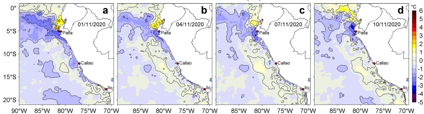
Figura 3. Anomalías de la temperatura superficial del mar (TSM, °C) para los días: a) 01, b) 04, c) 07 y d) 10 de noviembre de 2020. Las anomalías se calcularon respecto de la climatología para el periodo 2007-2016. Datos: OSTIA-UKMO-L4-GLOB-v2.0 (UK Met Office, 2012; Donlon et al, 2012). Procesamiento: LHF/AFIOF/DGIOCC.
