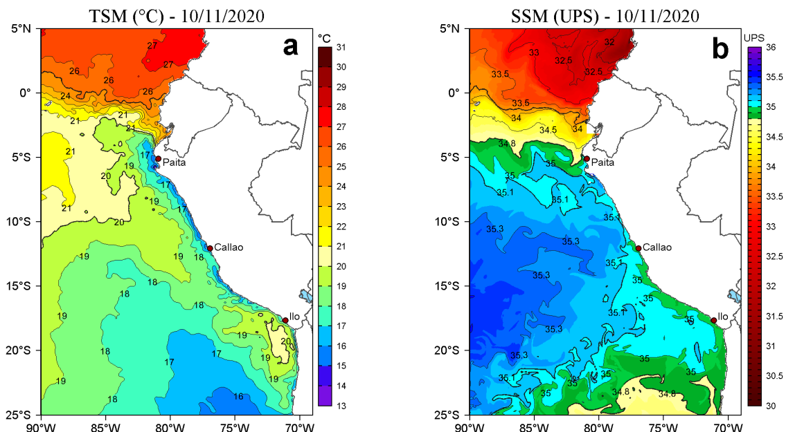
Figura 2. a) Temperatura superficial del mar (TSM, °C) y b) Salinidad superficial del mar (SSM, UPS), para el 10 de noviembre de 2020. Datos: OSTIA-UKMO-L4-GLOB-v2.0 (UK Met Office, 2012; Donlon et al, 2012) disponible en https://podaac.jpl.nasa.gov/dataset/OSTIA-UKMO-L4-GLOB-v2.0 para (a) y Hybrid Coordinate Ocean Model v. GOFS 3.1 (HYCOM; Halliwell et al., 1998; 2000; Bleck, 2001) para (b). Procesamiento: LHF/AFIOF/DGIOCC.
