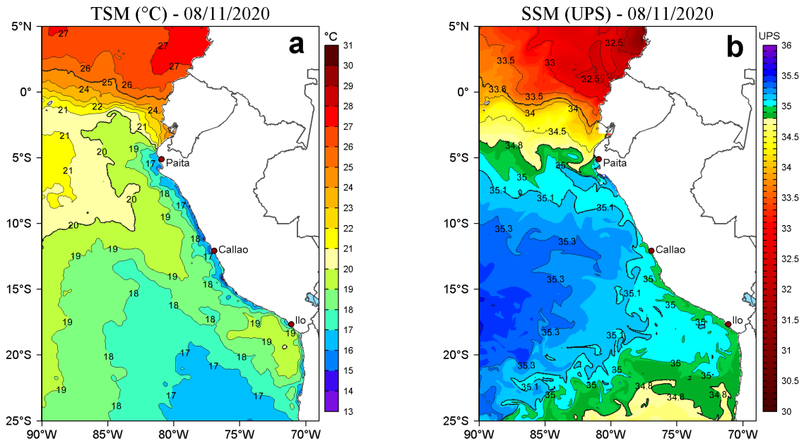
Figura 2. a) Temperatura superficial del mar (TSM, °C) y b) Salinidad superficial del mar (SSM, UPS), para el 08 de noviembre de 2020. Datos: OSTIA-UKMO-L4-GLOB-v2.0 (UK Met Office, 2012; Donlon et al, 2012) disponible en https://podaac.jpl.nasa.gov/dataset/OSTIA-UKMO-L4-GLOB-v2.0 para (a) y Hybrid Coordinate Ocean Model v. GOFS 3.1 (HYCOM; Halliwell et al., 1998; 2000; Bleck, 2001) para (b). Procesamiento: LHFMA/AFIOF/DGIOCC.
