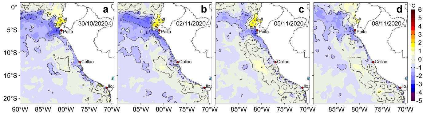
Figura 3. Anomalías de la temperatura superficial del mar (TSM, °C) para los días: a) 30 de octubre, b) 02, c) 05 y d) 08 de noviembre de 2020. Las anomalías se calcularon respecto de la climatología para el periodo 2007-2016. Datos: OSTIA-UKMO-L4-GLOB-v2.0 (UK Met Office, 2012; Donlon et al, 2012). Procesamiento: LHFMA/AFIOF/DGIOCC.
