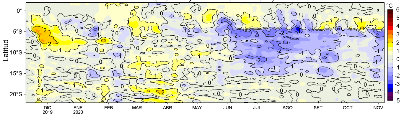
Figura 4. Variación promedio de las anomalías de la temperatura superficial del mar (TSM, °C) para una franja de 60 mn (~111 km) adyacente al litoral peruano para los últimos doce meses al 07 de noviembre de 2020. Datos: OSTIA-UKMO-L4-GLOB-v2.0 (UK Met. Office, 2012; Donlon et al, 2012) disponible en https://podaac.jpl.nasa.gov/dataset/OSTIA-UKMO-L4-GLOB-v2.0 . Las anomalías se calcularon con respecto al periodo 2007-2016. Procesamiento: LHFm/AFIOF/DGIOCC.
