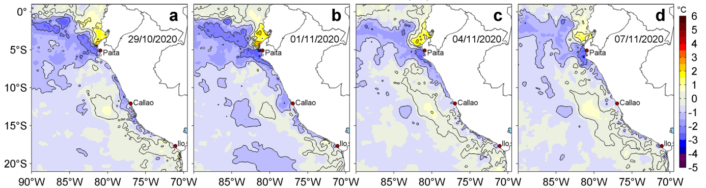
Figura 3. Anomalías de la temperatura superficial del mar (TSM, °C) para los días: a) 29 de octubre, b) 01, c) 04 y d) 07 de noviembre de 2020. Las anomalías se calcularon respecto de la climatología para el periodo 2007-2016. Datos: OSTIA-UKMO-L4-GLOB-v2.0 (UK Met Office, 2012; Donlon et al, 2012). Procesamiento: LHFm/AFIOF/DGIOCC.
