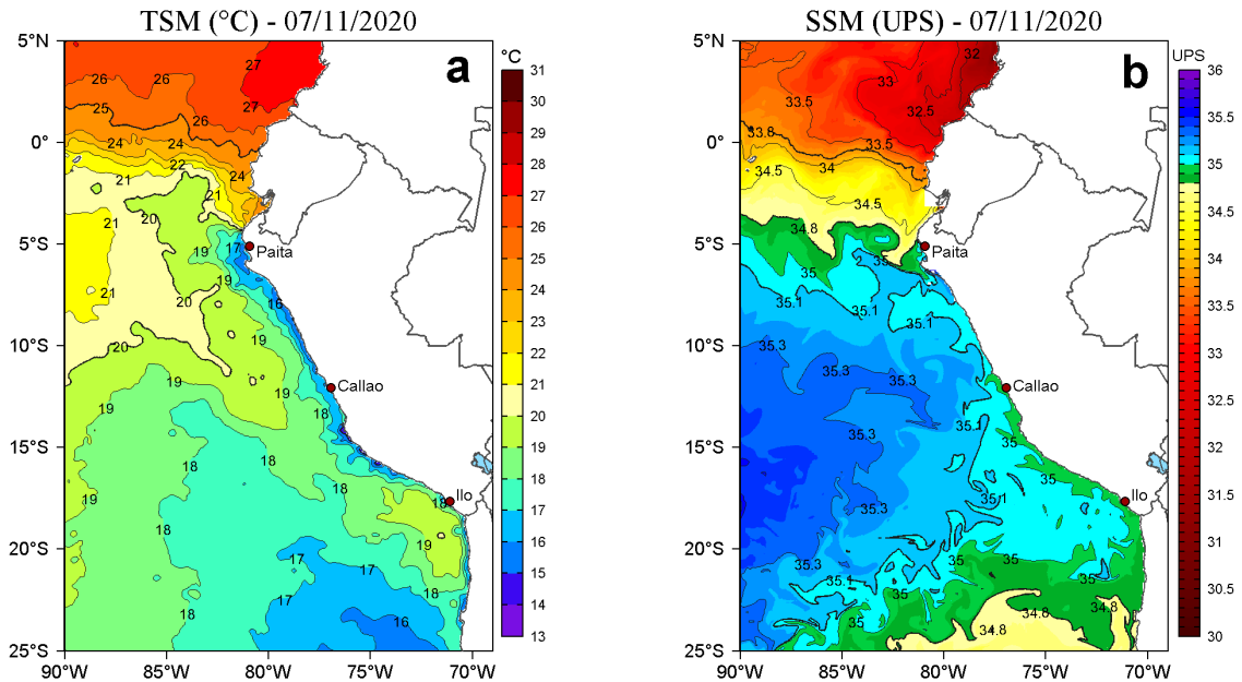
Figura 2. a) Temperatura superficial del mar (TSM, °C) y b) Salinidad superficial del mar (SSM, UPS), para el 07 de noviembre de 2020. Datos: OSTIA-UKMO-L4-GLOB-v2.0 (UK Met Office, 2012; Donlon et al, 2012) disponible en https://podaac.jpl.nasa.gov/dataset/OSTIA-UKMO-L4-GLOB-v2.0 para (a) y Hybrid Coordinate Ocean Model v. GOFS 3.1 (HYCOM; Halliwell et al., 1998; 2000; Bleck, 2001) para (b). Procesamiento: LHFm/AFIOF/DGIOCC.
