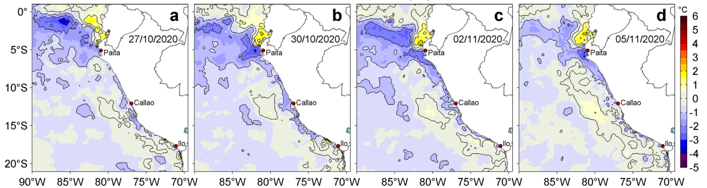
Figura 3. Anomalías de la temperatura superficial del mar (TSM, °C) para los días: a) 27 y b) 30 de octubre, c) 02 y d) 05 de noviembre de 2020. Las anomalías se calcularon respecto de la climatología para el periodo 2007-2016. Datos: OSTIA-UKMO-L4-GLOB-v2.0 (UK Met Office, 2012; Donlon et al, 2012). Procesamiento: LHF/AFIOF/DGIOCC.
