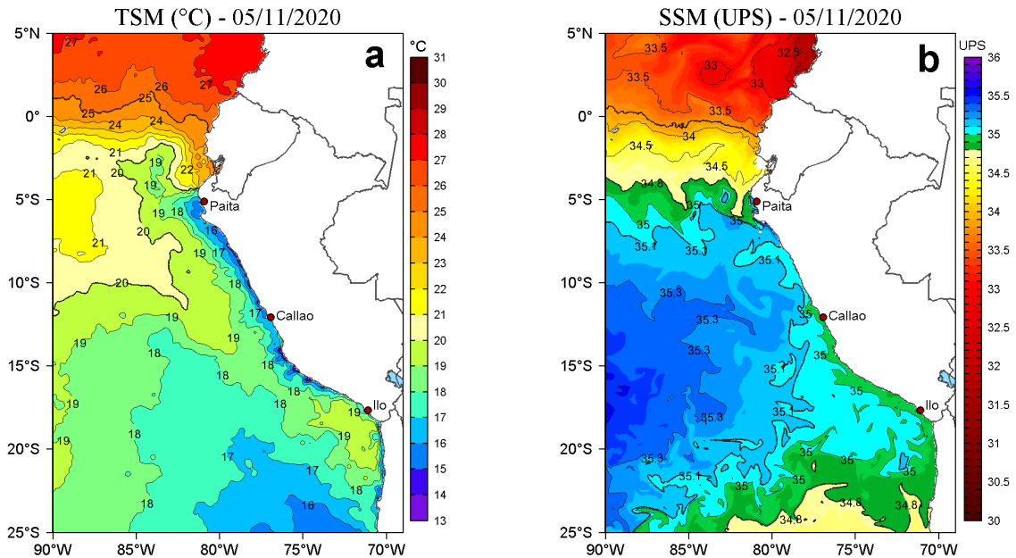
Figura 2. a) Temperatura superficial del mar (TSM, °C) y b) Salinidad superficial del mar (SSM, UPS), para el 05 de noviembre de 2020. Datos: OSTIA-UKMO-L4-GLOB-v2.0 (UK Met Office, 2012; Donlon et al, 2012) disponible en https://podaac.jpl.nasa.gov/dataset/OSTIA-UKMO-L4-GLOB-v2.0 para (a) y Hybrid Coordinate Ocean Model v. GOFS 3.1 (HYCOM; Halliwell et al., 1998; 2000; Bleck, 2001) para (b). Procesamiento: LHF/AFIOF/DGIOCC.
