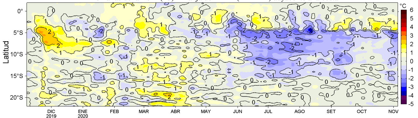
Figura 4. Variación promedio de las anomalías de la temperatura superficial del mar (TSM, °C) para una franja de 60 mn (~111 km) adyacente al litoral peruano para los últimos doce meses al 05 de noviembre de 2020. Datos: OSTIA-UKMO-L4-GLOB-v2.0 (UK Met. Office, 2012; Donlon et al, 2012) disponible en https://podaac.jpl.nasa.gov/dataset/OSTIA-UKMO-L4-GLOB-v2.0 . Las anomalías se calcularon con respecto al periodo 2007-2016. Procesamiento: LHF/AFIOF/DGIOCC.
