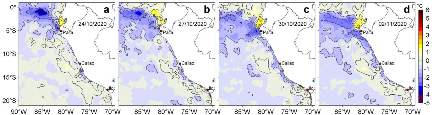
Figura 3. Anomalías de la temperatura superficial del mar (TSM, °C) para los días: a) 24, b) 27 y c) 30 de octubre y d) 02 de noviembre de 2020. Las anomalías se calcularon respecto de la climatología para el periodo 2007-2016. Datos: OSTIA-UKMO-L4-GLOB-v2.0 (UK Met Office, 2012; Donlon et al, 2012). Procesamiento: LHFMA/AFIOF/DGIOCC.
