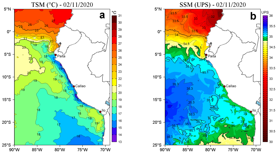
Figura 2. a) Temperatura superficial del mar (TSM, °C) y b) Salinidad superficial del mar (SSM, UPS), para el 02 de noviembre de 2020. Datos: OSTIA-UKMO-L4-GLOB-v2.0 (UK Met Office, 2012; Donlon et al, 2012) disponible en https://podaac.jpl.nasa.gov/dataset/OSTIA-UKMO-L4-GLOB-v2.0 para (a) y Hybrid Coordinate Ocean Model v. GOFS 3.1 (HYCOM; Halliwell et al., 1998; 2000; Bleck, 2001) para (b). Procesamiento: LHFMA/AFIOF/DGIOCC.
