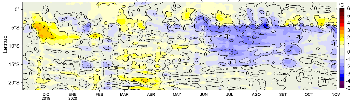
Figura 4. Variación promedio de las anomalías de la temperatura superficial del mar (TSM, °C) para una franja de 60 mn (~111 km) adyacente al litoral peruano para los últimos doce meses al 02 de noviembre de 2020. Datos: OSTIA-UKMO-L4-GLOB-v2.0 (UK Met. Office, 2012; Donlon et al, 2012) disponible en https://podaac.jpl.nasa.gov/dataset/OSTIA-UKMO-L4-GLOB-v2.0 . Las anomalías se calcularon con respecto al periodo 2007-2016. Procesamiento: LHFMA/AFIOF/DGIOCC.
