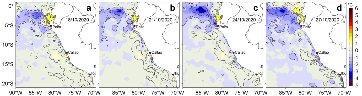
Figura 3. Anomalías de la temperatura superficial del mar (TSM, °C) para los días: a) 18, b) 21, c) 24 y d) 27 de octubre de 2020. Las anomalías se calcularon respecto de la climatología para el periodo 2007-2016. Datos: OSTIA-UKMO-L4-GLOB-v2.0 (UK Met Office, 2012; Donlon et al, 2012). Procesamiento: LHFm/AFIOF/DGIOCC.
