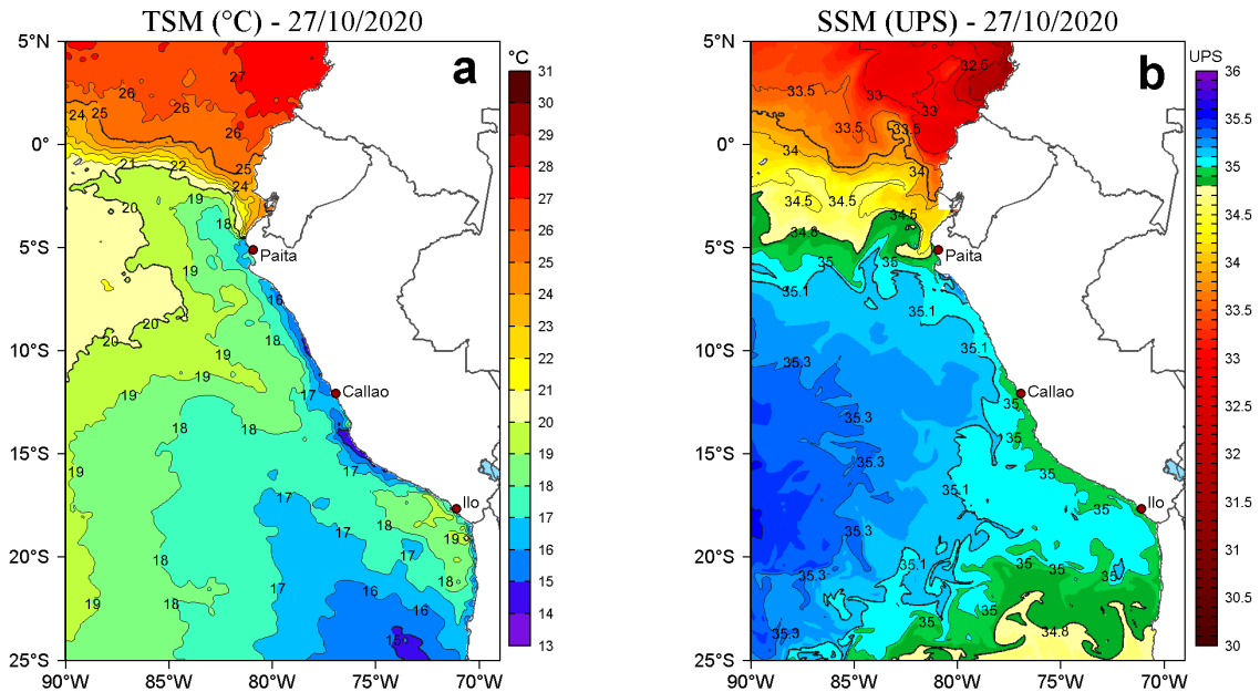
Figura 2. a) Temperatura superficial del mar (TSM, °C) y b) Salinidad superficial del mar (SSM, UPS), para el 27 de octubre de 2020. Datos: OSTIA-UKMO-L4-GLOB-v2.0 (UK Met Office, 2012; Donlon et al, 2012) disponible en https://podaac.jpl.nasa.gov/dataset/OSTIA-UKMO-L4-GLOB-v2.0 para (a) y Hybrid Coordinate Ocean Model v. GOFS 3.1 (HYCOM; Halliwell et al., 1998; 2000; Bleck, 2001) para (b). Procesamiento: LHFm/AFIOF/DGIOCC.
