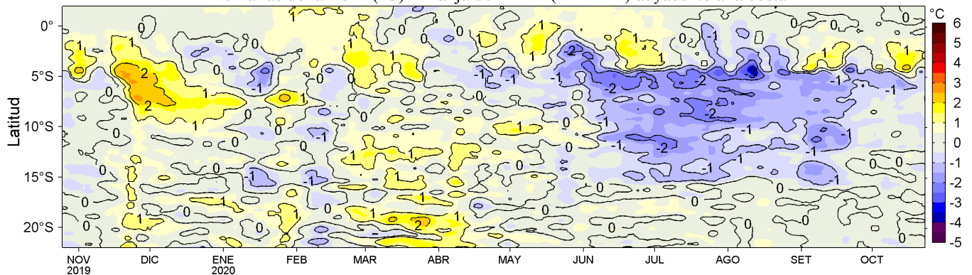
Figura 4. Variación promedio de las anomalías de la temperatura superficial del mar (TSM, °C) para una franja de 60 mn (~111 km) adyacente al litoral peruano para los últimos doce meses al 23 de octubre de 2020. Datos: OSTIA-UKMO-L4-GLOB-v2.0 (UK Met. Office, 2012; Donlon et al, 2012) disponible en https://podaac.jpl.nasa.gov/dataset/OSTIA-UKMO-L4-GLOB-v2.0 . Las anomalías se calcularon con respecto al periodo 2007-2016. Procesamiento: LHF/AFIOF/DGIOCC.
