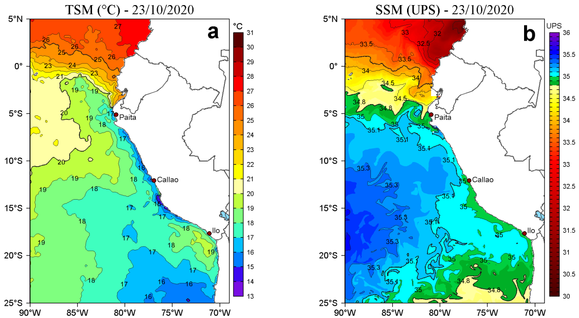
Figura 2. a) Temperatura superficial del mar (TSM, °C) y b) Salinidad superficial del mar (SSM, UPS), para el 23 de octubre de 2020. Datos: OSTIA-UKMO-L4-GLOB-v2.0 (UK Met Office, 2012; Donlon et al, 2012) disponible en https://podaac.jpl.nasa.gov/dataset/OSTIA-UKMO-L4-GLOB-v2.0 para (a) y Hybrid Coordinate Ocean Model v. GOF3 3.1 (HYCOM; Halliwell et al., 1998; 2000; Bleck, 2001) para (b). Procesamiento: LHF/AFIOF/DGIOCC.
