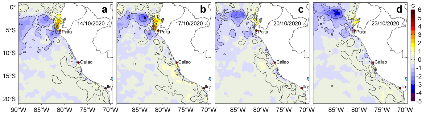
Figura 3. Anomalías de la temperatura superficial del mar (TSM, °C) para los días: a) 14, b) 17, c) 20 y d) 23 de octubre de 2020. Las anomalías se calcularon respecto de la climatología para el periodo 2007-2016. Datos: OSTIA-UKMO-L4-GLOB-v2.0 (UK Met Office, 2012; Donlon et al, 2012). Procesamiento: LHF/AFIOF/DGIOCC.
