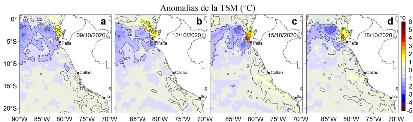
Figura 3. Anomalías de la temperatura superficial del mar (TSM, °C) para los días: a) 09, b) 12, c) 15 y d) 18 de octubre de 2020. Las anomalías se calcularon respecto de la climatología para el periodo 2007-2016. Datos: OSTIA-UKMO-L4-GLOB-v2.0 (UK Met Office, 2012; Donlon et al, 2012). Procesamiento: LHFM/AFIOF/DGIOCC.
