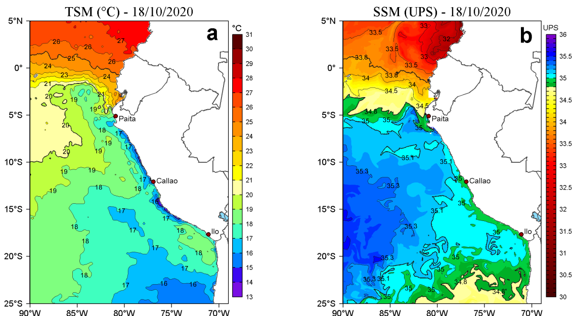
Figura 2. a) Temperatura superficial del mar (TSM, °C) y b) Salinidad superficial del mar (SSM, UPS), para el 18 de octubre de 2020. Datos: OSTIA-UKMO-L4-GLOB-v2.0 (UK Met Office, 2012; Donlon et al, 2012) disponible en https://podaac.jpl.nasa.gov/dataset/OSTIA-UKMO-L4-GLOB-v2.0 para (a) y Hybrid Coordinate Ocean Model v. GOFS 3.1 (HYCOM; Halliwell et al., 1998; 2000; Bleck, 2001) para (b). Procesamiento: LHFM/AFIOF/DGIOCC.
