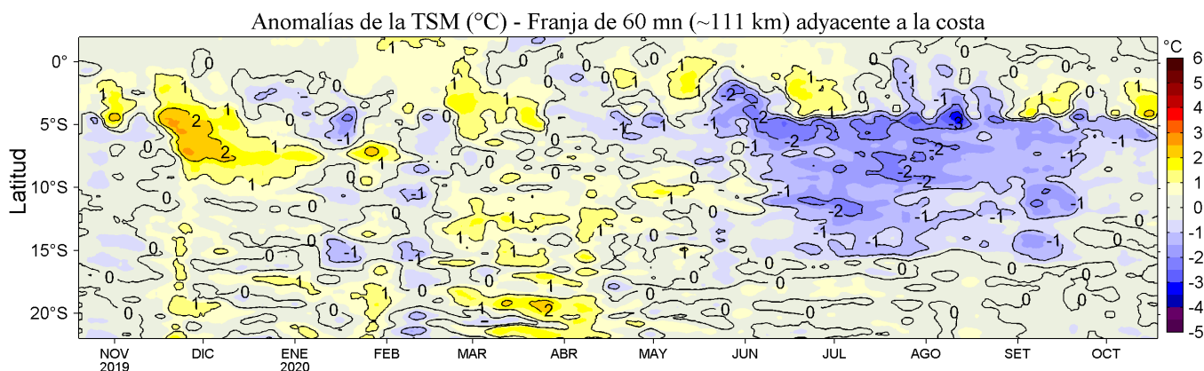
Figura 4. Variación promedio de las anomalías de la temperatura superficial del mar (TSM, °C) para una franja de 60 mn (~111 km) adyacente al litoral peruano para los últimos doce meses al 18 de octubre de 2020. Datos: OSTIA-UKMO-L4-GLOB-v2.0 (UK Met. Office, 2012; Donlon et al, 2012) disponible en https://podaac.jpl.nasa.gov/dataset/OSTIA-UKMO-L4-GLOB-v2.0 . Las anomalías se calcularon con respecto al periodo 2007-2016. Procesamiento: LHFM/AFIOF/DGIOCC.
