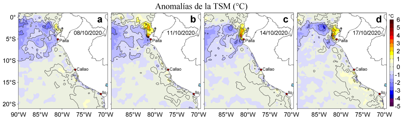
Figura 3. Anomalías de la temperatura superficial del mar (TSM, °C) para los días: a) 08, b) 11, c) 14 y d) 17 de octubre de 2020. Las anomalías se calcularon respecto de la climatología para el periodo 2007-2016. Datos: OSTIA-UKMO-L4-GLOB-v2.0 (UK Met Office, 2012; Donlon et al, 2012). Procesamiento: LHFM/AFIOF/DGIOCC.
