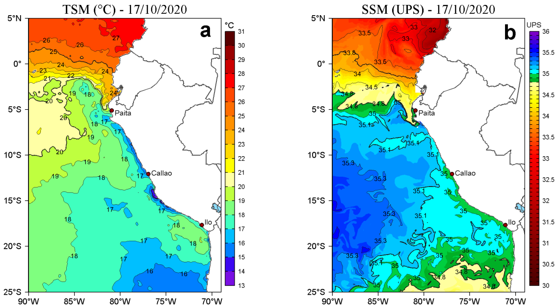
Figura 2. a) Temperatura superficial del mar (TSM, °C) y b) Salinidad superficial del mar (SSM, UPS), para el 17 de octubre de 2020. Datos: OSTIA-UKMO-L4-GLOB-v2.0 (UK Met Office, 2012; Donlon et al, 2012) disponible en https://podaac.jpl.nasa.gov/dataset/OSTIA-UKMO-L4-GLOB-v2.0 para (a) y Hybrid Coordinate Ocean Model v. GOFS 3.1 (HYCOM; Halliwell et al., 1998; 2000; Bleck, 2001) para (b). Procesamiento: LHFM/AFIOF/DGIOCC.
