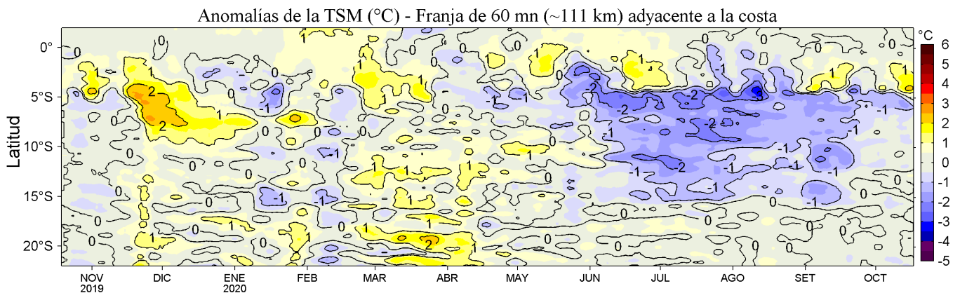
Figura 4. Variación promedio de las anomalías de la temperatura superficial del mar (TSM, °C) para una franja de 60 mn (~111 km) adyacente al litoral peruano para los últimos doce meses al 17 de octubre de 2020. Datos: OSTIA-UKMO-L4-GLOB-v2.0 (UK Met. Office, 2012; Donlon et al, 2012) disponible en https://podaac.jpl.nasa.gov/dataset/OSTIA-UKMO-L4-GLOB-v2.0 . Las anomalías se calcularon con respecto al periodo 2007-2016. Procesamiento: LHFM/AFIOF/DGIOCC.
