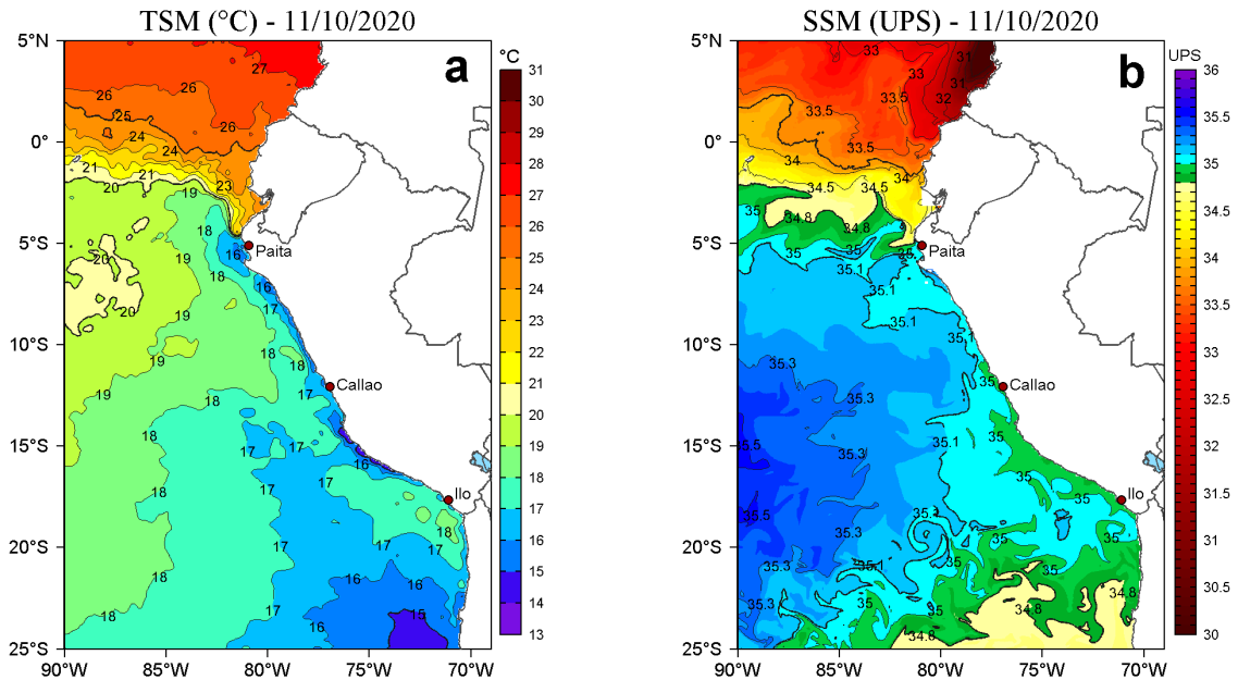
Figura 2. a) Temperatura superficial del mar (TSM, °C) y b) Salinidad superficial del mar (SSM, UPS), para el 11 de octubre de 2020. Datos: OSTIA-UKMO-L4-GLOB-v2.0 (UK Met Office, 2012; Donlon et al, 2012) disponible en https://podaac.jpl.nasa.gov/dataset/OSTIA-UKMO-L4-GLOB-v2.0 para (a) y Hybrid Coordinate Ocean Model v. GOFS 3.1 (HYCOM; Halliwell et al., 1998; 2000; Bleck, 2001) para (b). Procesamiento: LHFm/AFIOF/DGIOCC.
