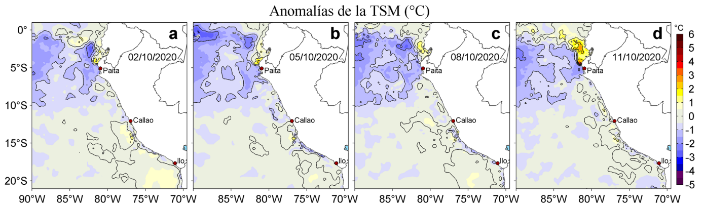
Figura 3. Anomalías de la temperatura superficial del mar (TSM, °C) para los días: a) 02, b) 05, c) 08 y d) 11 de octubre de 2020. Las anomalías se calcularon respecto de la climatología para el periodo 2007-2016. Datos: OSTIA-UKMO-L4-GLOB-v2.0 (UK Met Office, 2012; Donlon et al, 2012). Procesamiento: LHFm/AFIOF/DGIOCC.
