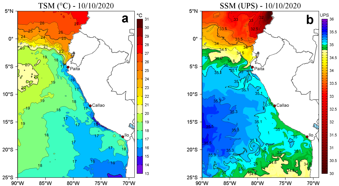
Figura 2. a) Temperatura superficial del mar (TSM, °C) y b) Salinidad superficial del mar (SSM, UPS), para el 10 de octubre de 2020. Datos: OSTIA-UKMO-L4-GLOB-v2.0 (UK Met Office, 2012; Donlon et al, 2012) disponible en https://podaac.jpl.nasa.gov/dataset/OSTIA-UKMO-L4-GLOB-v2.0 para (a) y Hybrid Coordinate Ocean Model v. GOFS 3.1 (HYCOM; Halliwell et al., 1998; 2000; Bleck, 2001) para (b). Procesamiento: LHF/AFIOF/DGIOCC.
