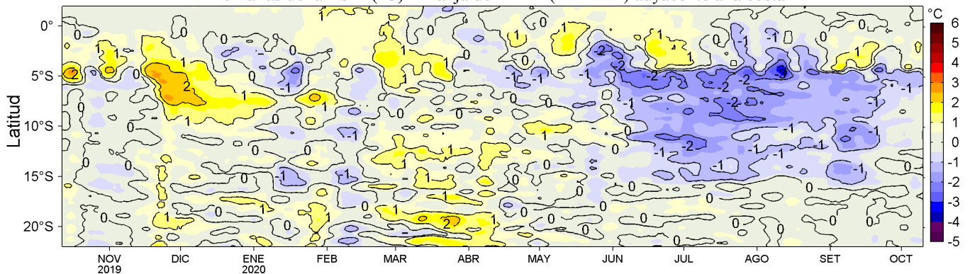
Figura 4. Variación promedio de las anomalías de la temperatura superficial del mar (TSM, °C) para una franja de 60 mn (~111 km) adyacente al litoral peruano para los últimos doce meses al 10 de octubre de 2020. Datos: OSTIA-UKMO-L4-GLOB-v2.0 (UK Met. Office, 2012; Donlon et al, 2012) disponible en https://podaac.jpl.nasa.gov/dataset/OSTIA-UKMO-L4-GLOB-v2.0 . Las anomalías se calcularon con respecto al periodo 2007-2016. Procesamiento: LHF/AFIOF/DGIOCC.
