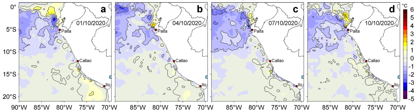
Figura 3. Anomalías de la temperatura superficial del mar (TSM, °C) para los días: a) 01, b) 04, c) 07 y d) 10 de octubre de 2020. Las anomalías se calcularon respecto de la climatología para el periodo 2007-2016. Datos: OSTIA-UKMO-L4-GLOB-v2.0 (UK Met Office, 2012; Donlon et al, 2012). Procesamiento: LHF/AFIOF/DGIOCC.
