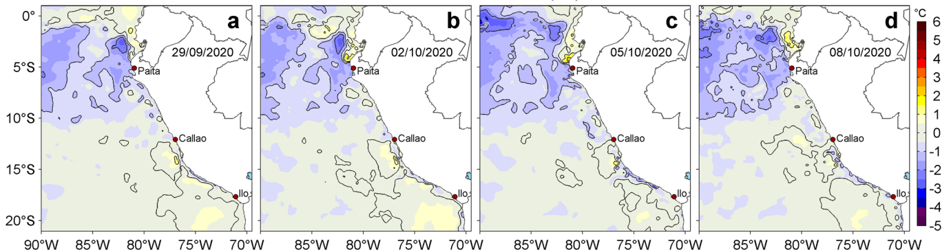
Figura 3. Anomalías de la temperatura superficial del mar (TSM, °C) para los días: a) 29 de setiembre, b) 02, c) 05 y d) 08 de octubre de 2020. Las anomalías se calcularon respecto de la climatología para el periodo 2007-2016. Datos: OSTIA-UKMO-L4-GLOB-v2.0 (UK Met Office, 2012; Donlon et al, 2012). Procesamiento: LHFH/AFIOF/DGIOCC.
