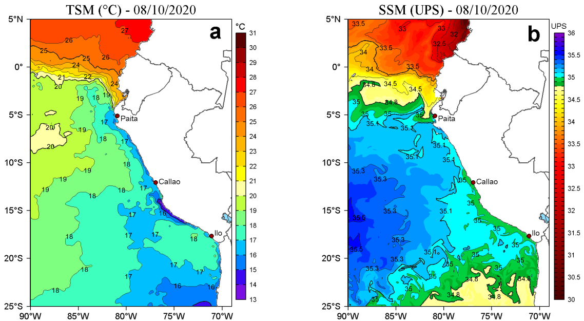
Figura 2. a) Temperatura superficial del mar (TSM, °C) y b) Salinidad superficial del mar (SSM, UPS), para el 08 de octubre de 2020. Datos: OSTIA-UKMO-L4-GLOB-v2.0 (UK Met Office, 2012; Donlon et al, 2012) disponible en https://podaac.jpl.nasa.gov/dataset/OSTIA-UKMO-L4-GLOB-v2.0 para (a) y Hybrid Coordinate Ocean Model v. GOFS 3.1 (HYCOM; Halliwell et al., 1998; 2000; Bleck, 2001) para (b). Procesamiento: LHFH/AFIOF/DGIOCC.
