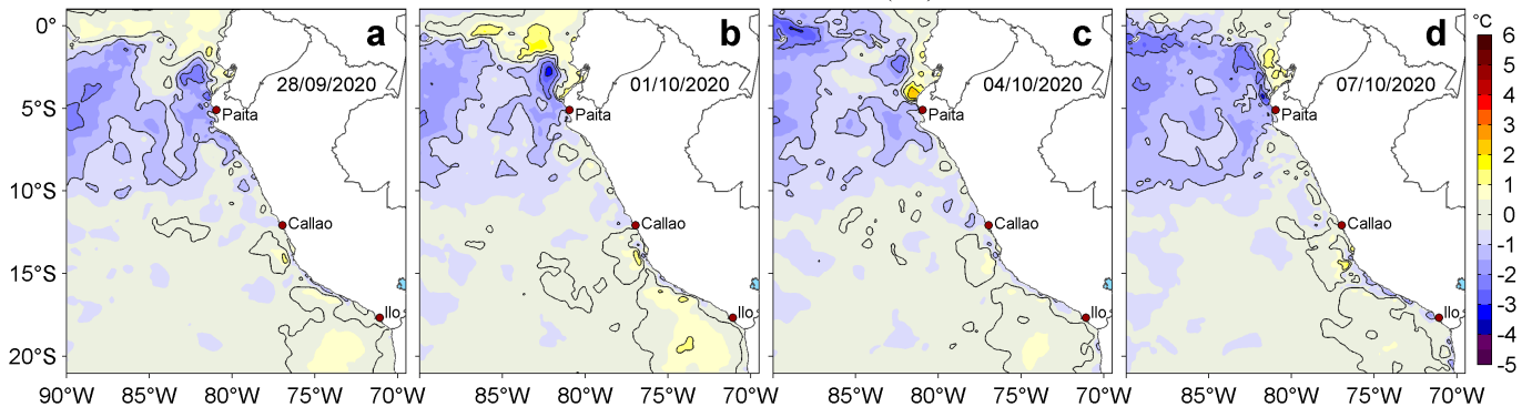
Figura 3. Anomalías de la temperatura superficial del mar (TSM, °C) para los días: a) 28 de setiembre, b) 01, c) 04 y d) 07 de octubre de 2020. Las anomalías se calcularon respecto de la climatología para el periodo 2007-2016. Datos: OSTIA-UKMO-L4-GLOB-v2.0 (UK Met Office, 2012; Donlon et al, 2012). Procesamiento: LHF/AFIOF/DGIOCC.
