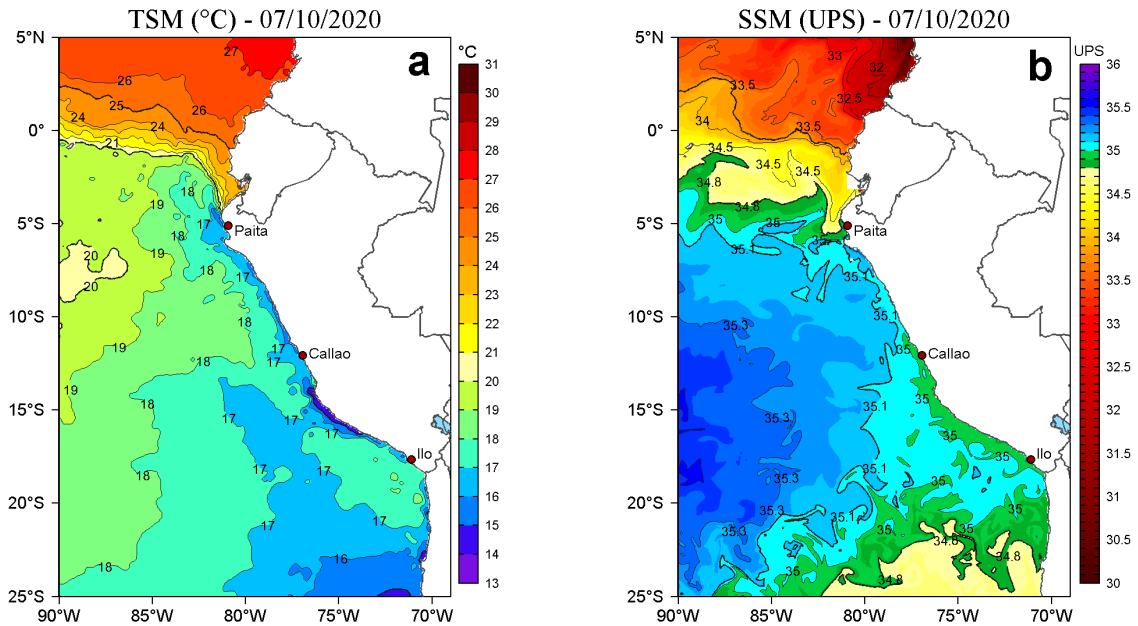
Figura 2. a) Temperatura superficial del mar (TSM, °C) y b) Salinidad superficial del mar (SSM, UPS), para el 07 de octubre de 2020. Datos: OSTIA-UKMO-L4-GLOB-v2.0 (UK Met Office, 2012; Donlon et al, 2012) disponible en https://podaac.jpl.nasa.gov/dataset/OSTIA-UKMO-L4-GLOB-v2.0 para (a) y Hybrid Coordinate Ocean Model v. GOF3 3.1 (HYCOM; Halliwell et al., 1998; 2000; Bleck, 2001) para (b). Procesamiento: LHF/AFIOF/DGIOCC.
