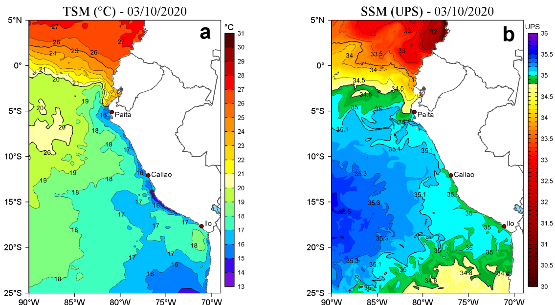
Figura 2. a) Temperatura superficial del mar (TSM, °C) y b) Salinidad superficial del mar (SSM, UPS), para el 03 de octubre de 2020. Datos: OSTIA-UKMO-L4-GLOB-v2.0 (UK Met Office, 2012; Donlon et al, 2012) disponible en https://podaac.jpl.nasa.gov/dataset/OSTIA-UKMO-L4-GLOB-v2.0 para (a) y Hybrid Coordinate Ocean Model v. GOFS 3.1 (HYCOM; Halliwell et al., 1998; 2000; Bleck, 2001) para (b). Procesamiento: LHFM/AFIOF/DGIOCC.
