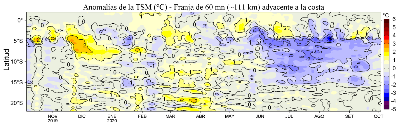
Figura 4. Variación promedio de las anomalías de la temperatura superficial del mar (TSM, °C) para una franja de 60 mn (~111 km) adyacente al litoral peruano para los últimos doce meses al 03 de octubre de 2020. Datos: OSTIA-UKMO-L4-GLOB-v2.0 (UK Met. Office, 2012; Donlon et al, 2012) disponible en https://podaac.jpl.nasa.gov/dataset/OSTIA-UKMO-L4-GLOB-v2.0 . Las anomalías se calcularon con respecto al periodo 2007-2016. Procesamiento: LHFM/AFIOF/DGIOCC.
