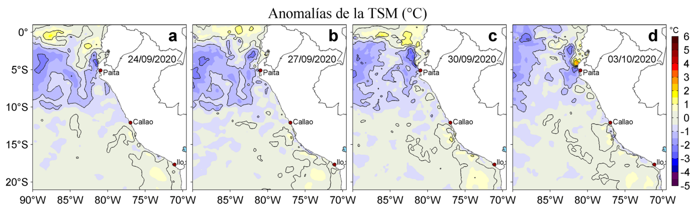
Figura 3. Anomalías de la temperatura superficial del mar (TSM, °C) para los días: a) 24, b) 27 y c) 30 de septiembre y d) 03 de octubre de 2020. Las anomalías se calcularon respecto de la climatología para el periodo 2007-2016. Datos: OSTIA-UKMO-L4-GLOB-v2.0 (UK Met Office, 2012; Donlon et al, 2012). Procesamiento: LHFM/AFIOF/DGIOCC.
