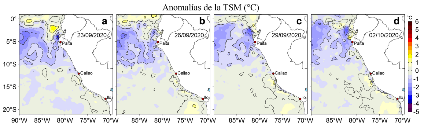
Figura 3. Anomalías de la temperatura superficial del mar (TSM, °C) para los días: a) 23, b) 26 y c) 29 de setiembre y d) 02 de octubre de 2020. Las anomalías se calcularon respecto de la climatología para el periodo 2007-2016. Datos: OSTIA-UKMO-L4-GLOB-v2.0 (UK Met Office, 2012; Donlon et al, 2012). Procesamiento: LHF/AFIOF/DGIOCC.
