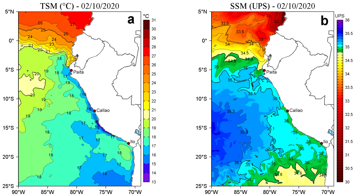
Figura 2. a) Temperatura superficial del mar (TSM, °C) y b) Salinidad superficial del mar (SSM, UPS), para el 02 de octubre de 2020. Datos: OSTIA-UKMO-L4-GLOB-v2.0 (UK Met Office, 2012; Donlon et al, 2012) disponible en https://podaac.jpl.nasa.gov/dataset/OSTIA-UKMO-L4-GLOB-v2.0 para (a) y Hybrid Coordinate Ocean Model v. GOFS 3.1 (HYCOM; Halliwell et al., 1998; 2000; Bleck, 2001) para (b). Procesamiento: LHF/AFIOF/DGIOCC.
