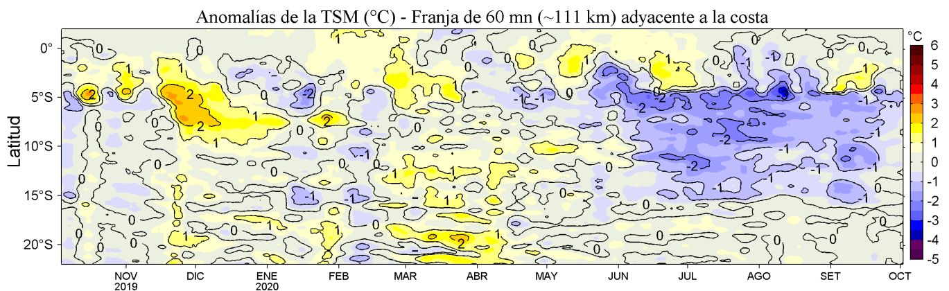
Figura 4. Variación promedio de las anomalías de la temperatura superficial del mar (TSM, °C) para una franja de 60 mn (~111 km) adyacente al litoral peruano para los últimos doce meses al 02 de octubre de 2020. Datos: OSTIA-UKMO-L4-GLOB-v2.0 (UK Met. Office, 2012; Donlon et al, 2012) disponible en https://podaac.jpl.nasa.gov/dataset/OSTIA-UKMO-L4-GLOB-v2.0 . Las anomalías se calcularon con respecto al periodo 2007-2016. Procesamiento: LHF/AFIOF/DGIOCC.
