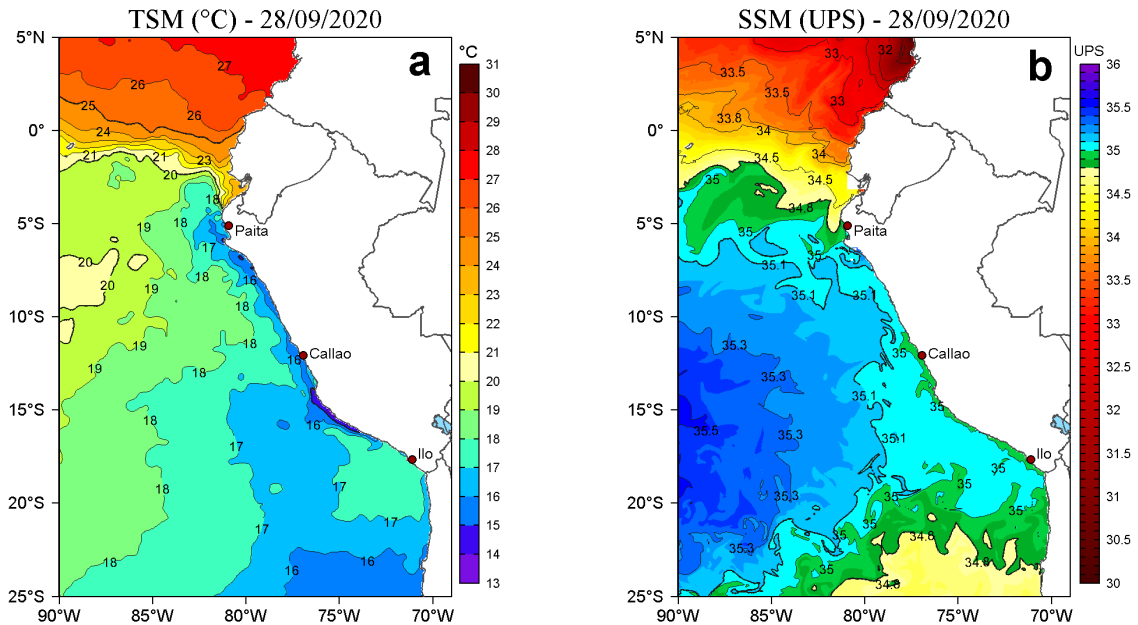
Figura 2. a) Temperatura superficial del mar (TSM, °C) y b) Salinidad superficial del mar (SSM, UPS), para el 28 de setiembre de 2020. Datos: OSTIA-UKMO-L4-GLOB-v2.0 (UK Met Office, 2012; Donlon et al, 2012) disponible en https://podaac.jpl.nasa.gov/dataset/OSTIA-UKMO-L4-GLOB-v2.0 para (a) y Hybrid Coordinate Ocean Model v. GOFS 3.1 (HYCOM; Halliwell et al., 1998; 2000; Bleck, 2001) para (b). Procesamiento: LHF/AFIOF/DGIOCC.
