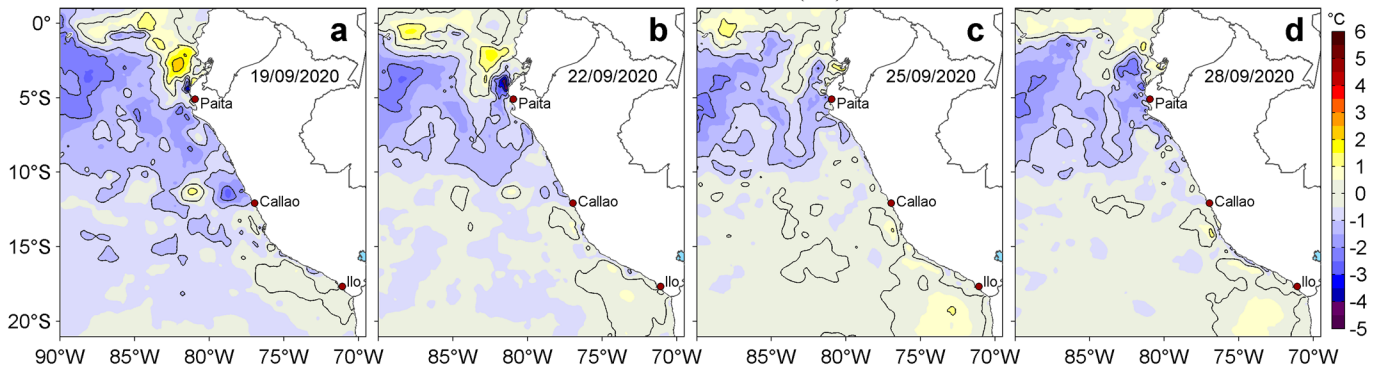
Figura 3. Anomalías de la temperatura superficial del mar (TSM, °C) para los días: a) 19, b) 22, c) 25 y d) 28 de setiembre de 2020. Las anomalías se calcularon respecto de la climatología para el periodo 2007-2016. Datos: OSTIA-UKMO-L4-GLOB-v2.0 (UK Met Office, 2012; Donlon et al, 2012). Procesamiento: LHF/AFIOF/DGIOCC.
