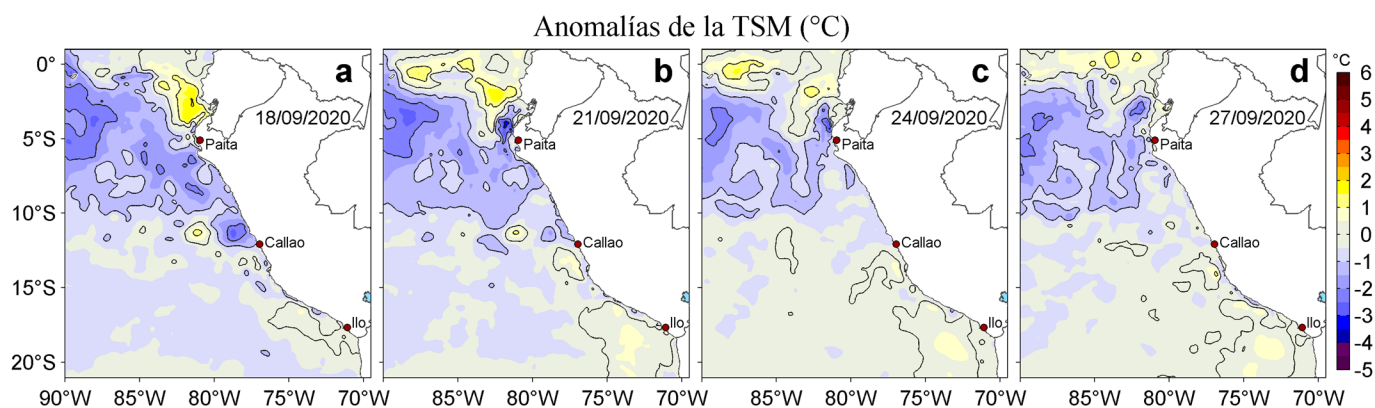
Figura 3. Anomalías de la temperatura superficial del mar (TSM, °C) para los días: a) 18, b) 21, c) 24 y d) 27 de setiembre de 2020. Las anomalías se calcularon respecto de la climatología para el periodo 2007-2016. Datos: OSTIA-UKMO-L4-GLOB-v2.0 (UK Met Office, 2012; Donlon et al, 2012). Procesamiento: LHF/AFIOF/DGIOCC.
