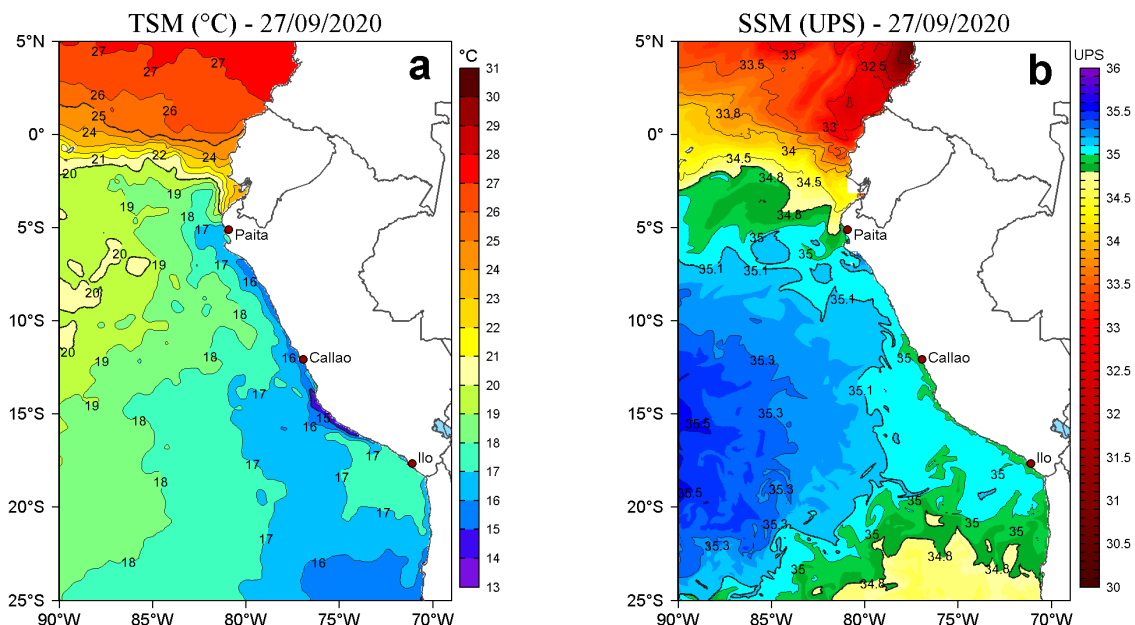
Figura 2. a) Temperatura superficial del mar (TSM, °C) y b) Salinidad superficial del mar (SSM, UPS), para el 27 de setiembre de 2020. Datos: OSTIA-UKMO-L4-GLOB-v2.0 (UK Met Office, 2012; Donlon et al, 2012) disponible en https://podaac.jpl.nasa.gov/dataset/OSTIA-UKMO-L4-GLOB-v2.0 para (a) y Hybrid Coordinate Ocean Model v. GOFS 3.1 (HYCOM; Halliwell et al., 1998; 2000; Bleck, 2001) para (b). Procesamiento: LHF/AFIOF/DGIOCC.
