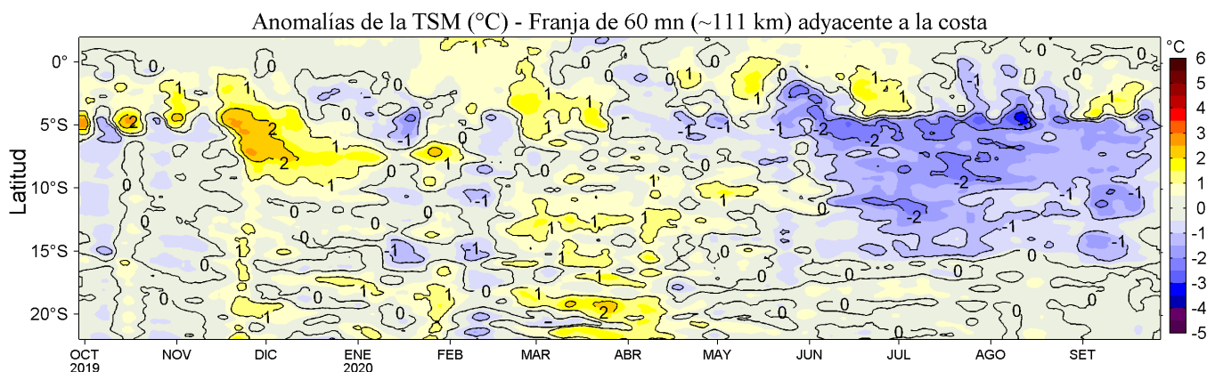
Figura 4. Variación promedio de las anomalías de la temperatura superficial del mar (TSM, °C) para una franja de 60 mn (~111 km) adyacente al litoral peruano para los últimos doce meses al 27 de setiembre de 2020. Datos: OSTIA-UKMO-L4-GLOB-v2.0 (UK Met. Office, 2012; Donlon et al, 2012) disponible en https://podaac.jpl.nasa.gov/dataset/OSTIA-UKMO-L4-GLOB-v2.0 . Las anomalías se calcularon con respecto al periodo 2007-2016. Procesamiento: LHF/AFIOF/DGIOCC.
